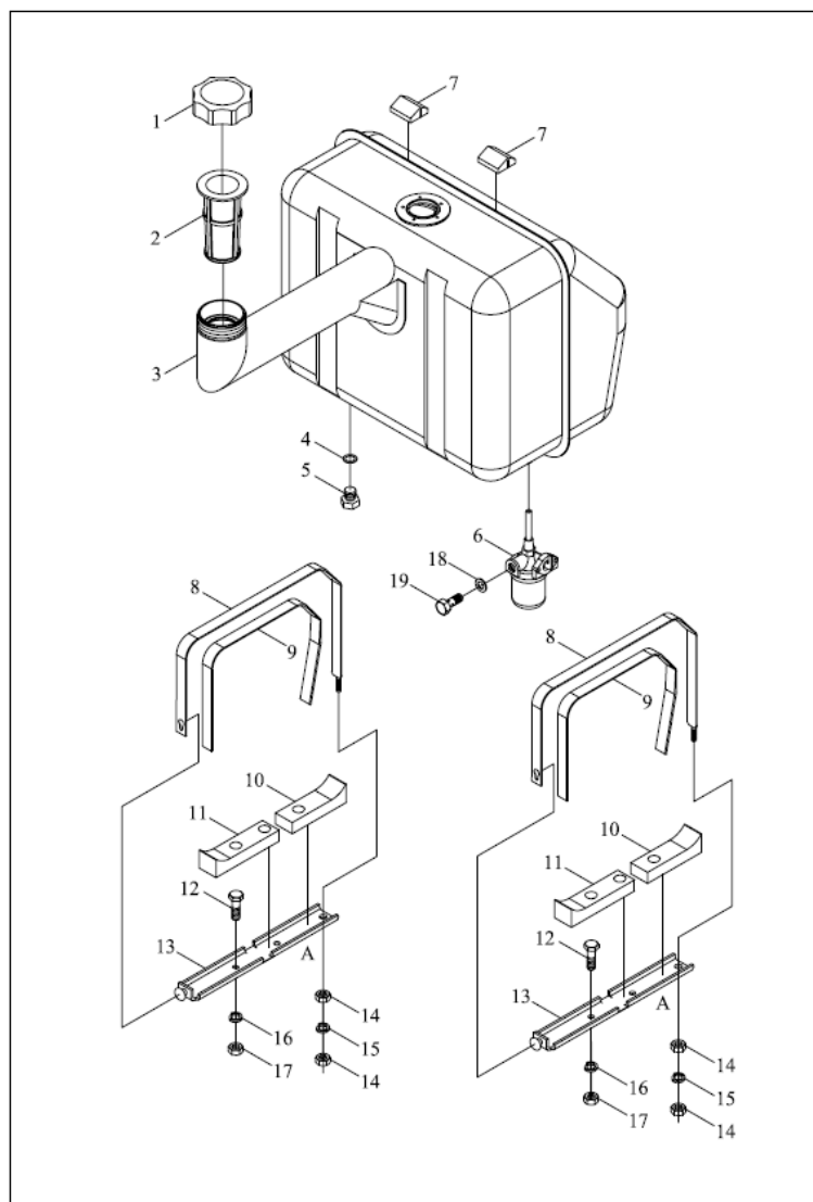
TB400.50X 燃油箱装配总成
