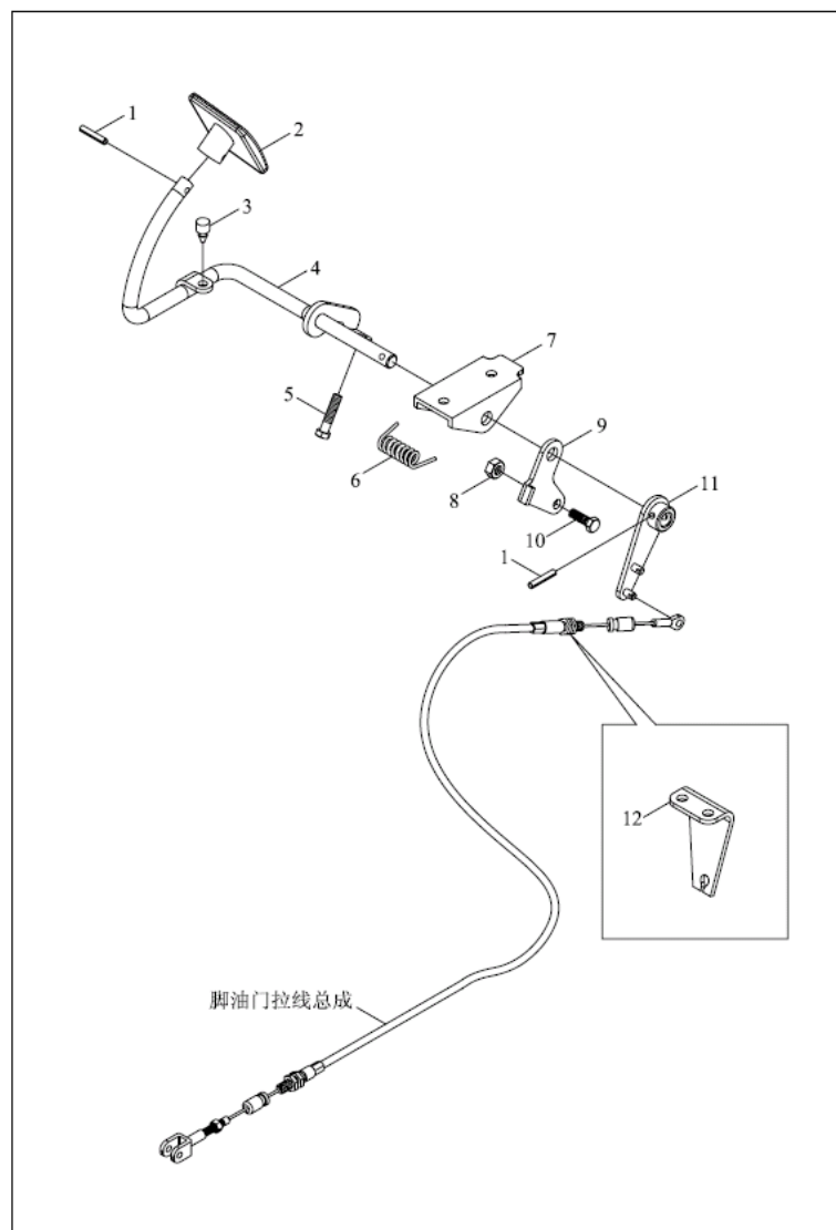
TB400.202B 脚油门总成
