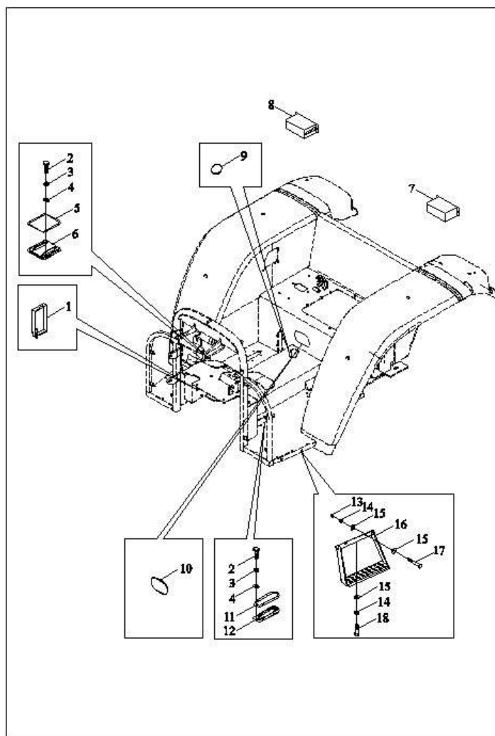
TB550.452U 地板总成-2
