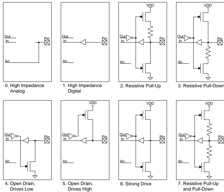
图 6-11. 驱动模式
