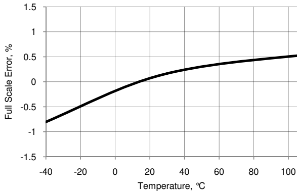
图 11-53. IDAC 全量程误差与温度, 范围 = 255 \mu\text{A} , 源电流模式
