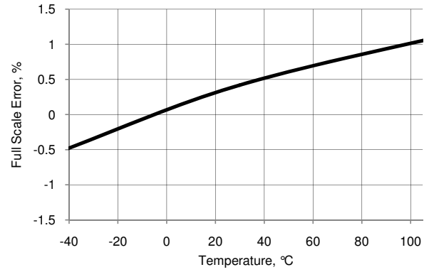
图 11-54. IDAC 全量程误差与温度, 范围 = 255 \mu\text{A} , 灌电流模式
