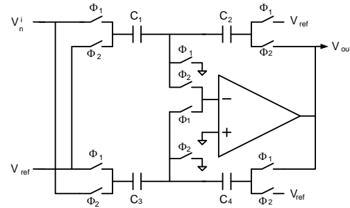
图 8-14. 采样和保持拓扑（Φ1 和 Φ2 是时钟的两个对立相位）
