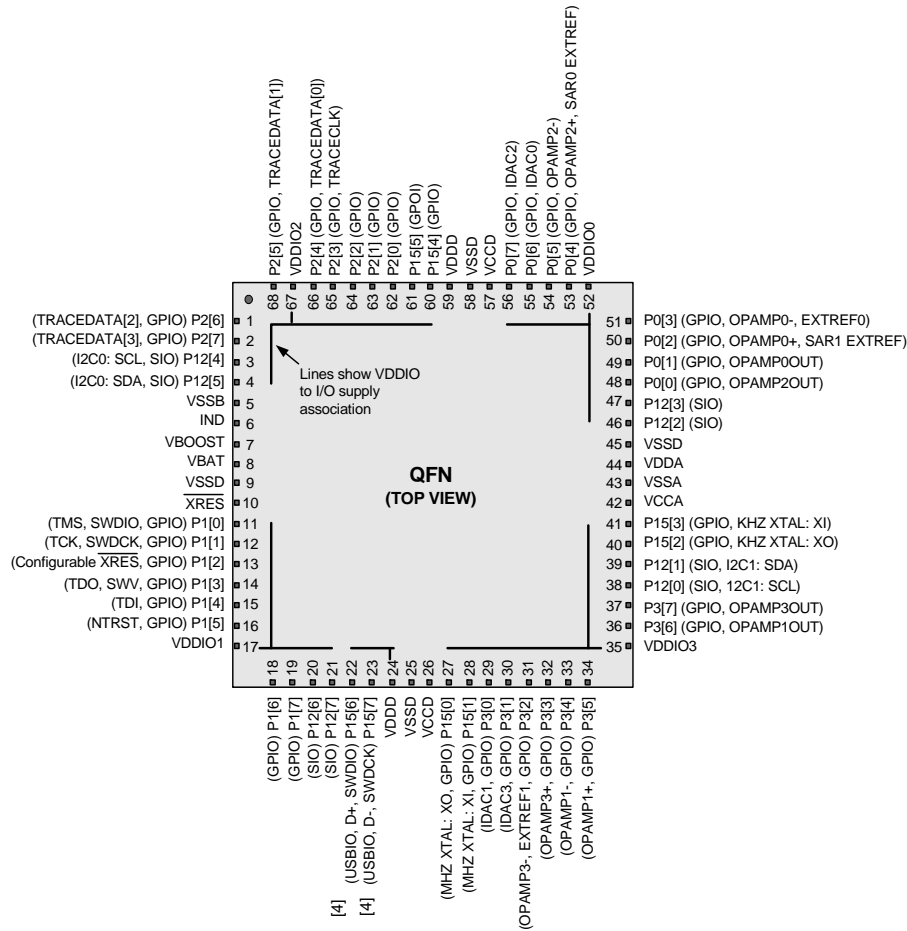
图 2-3. 68-QFN 器件的引脚分布 [3]
