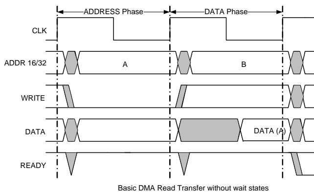
图 4-2. DMA 时序图
