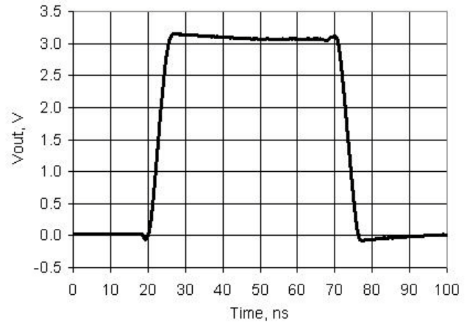
图 11-23. USBIO 输出上升和下降时间，GPIO 模式， V_{DD} = 3.3\text{ V} ， 25\text{ pF} 负载
