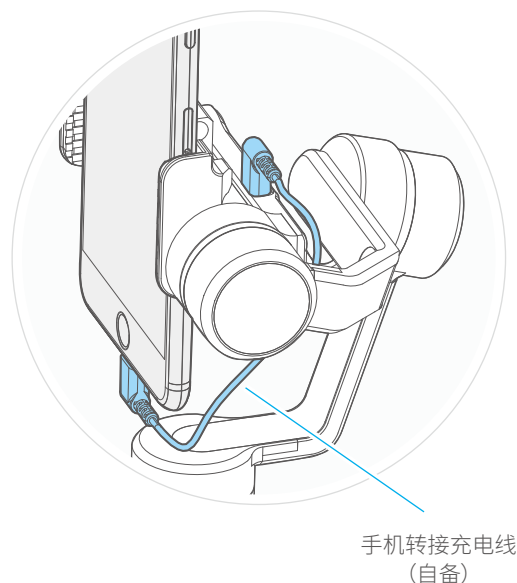
手机充电连接示意图
