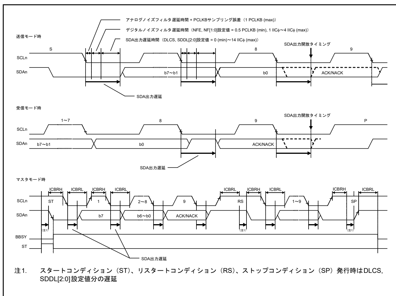
図 30.22 SDA 出力遅延機能
