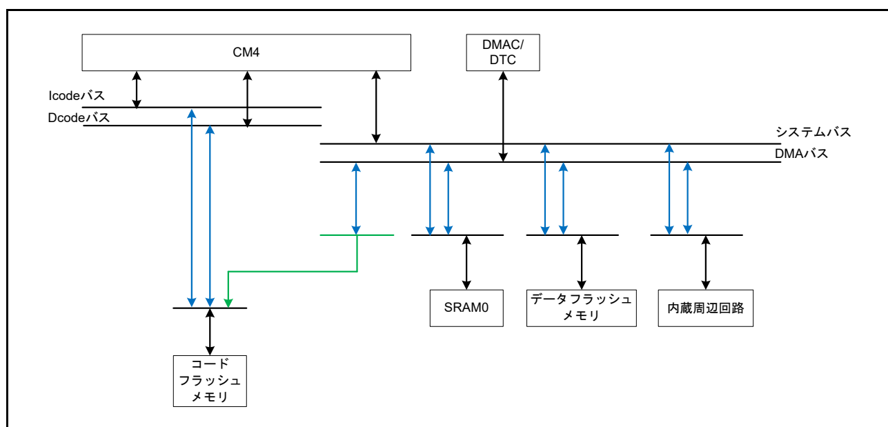
図 15.1 バスの構成図
