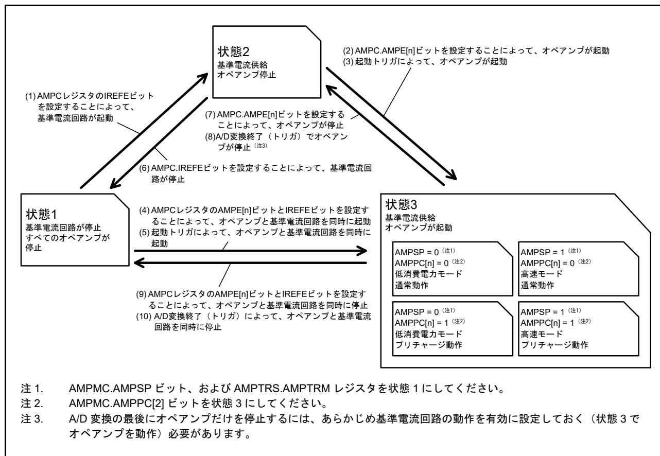
図 37.2 オペアンプの状態遷移
