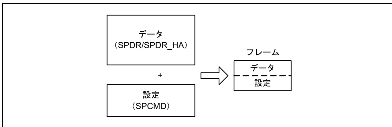
図 32.55 マスタモードでのシリアル転送フォーマットの決定方法 (SPI1)
