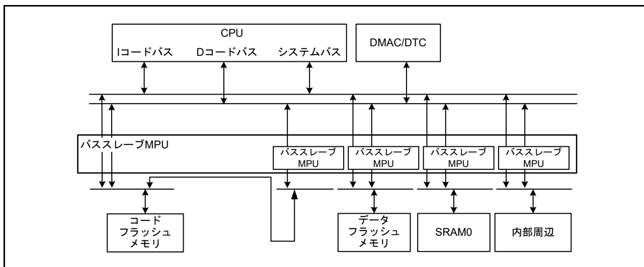
図 16.9 バススレーブ MPU のブロック図
