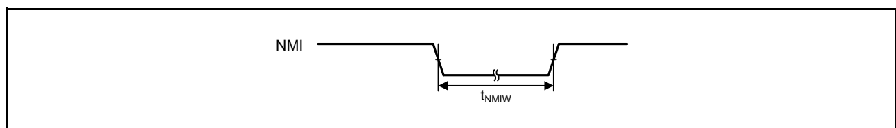
図 48.33 NMI 割り込み入力タイミング
