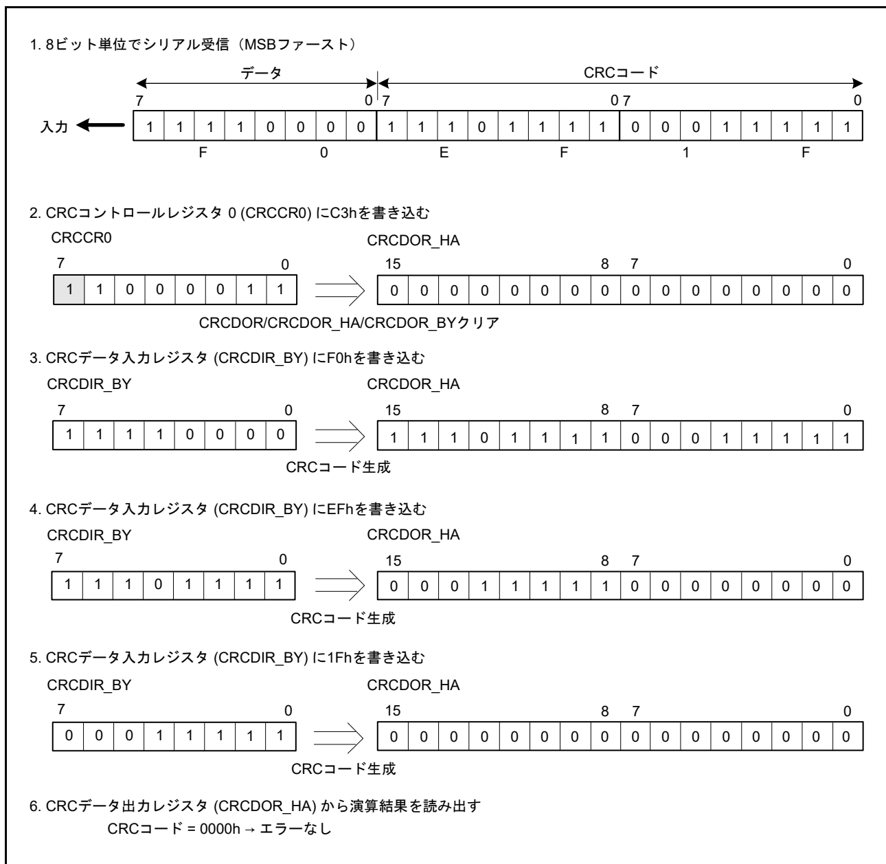
図 33.5 MSB ファーストのデータ受信
