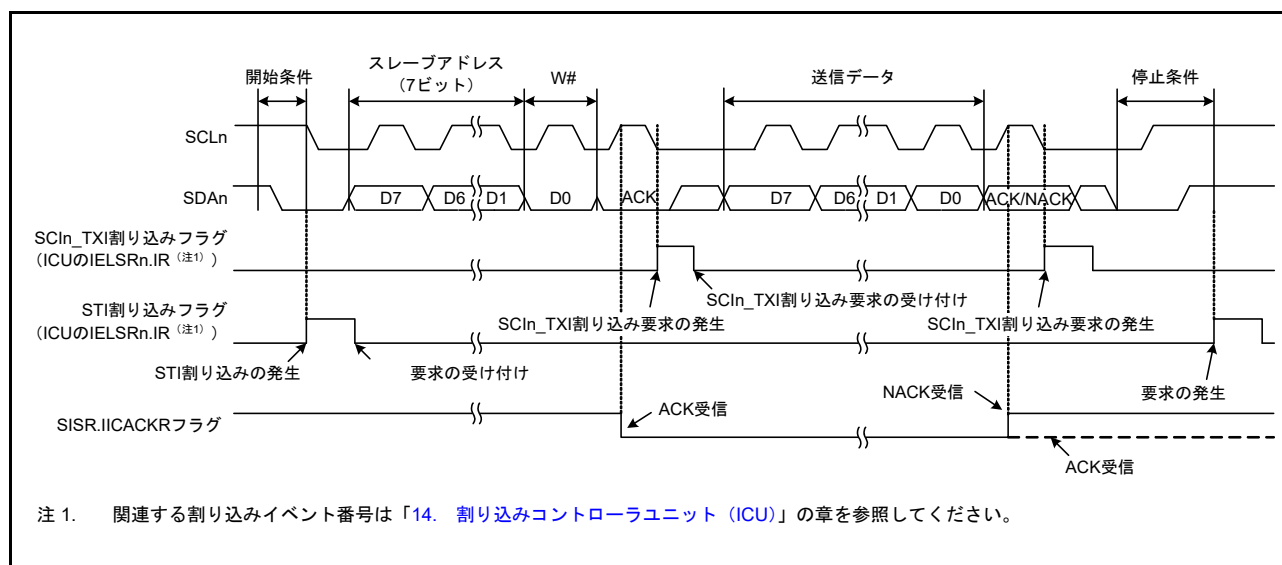
図 29.64 簡易 IIC モードにおけるマスタ送信の動作例 1 (7 ビットスレーブアドレス、送信割り込み、受信割り込み使用時)
