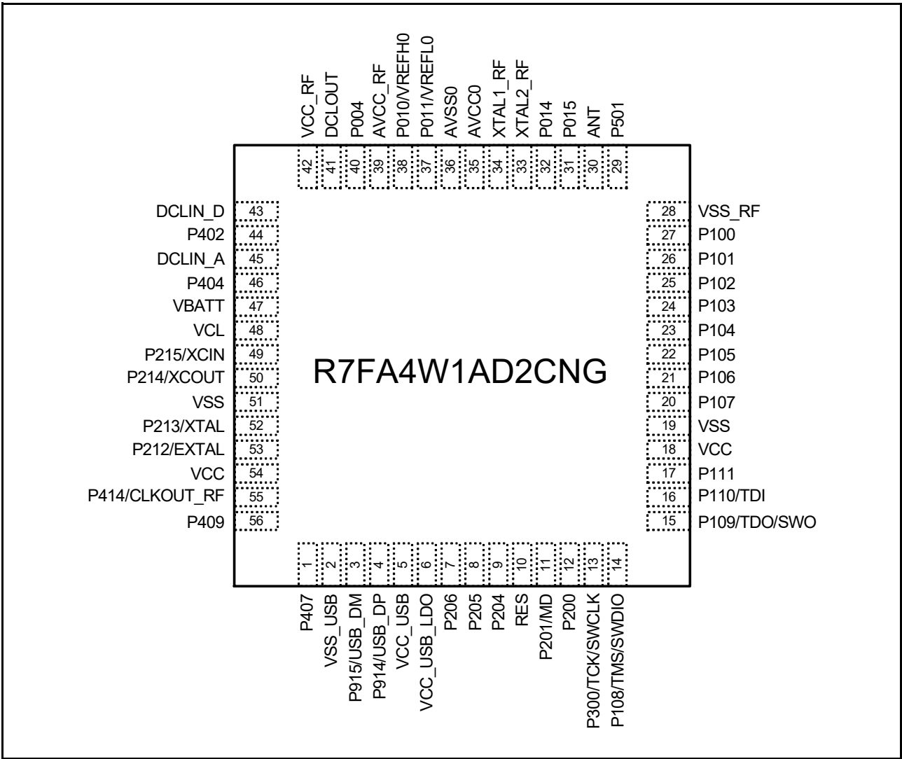
図 1.3 56-pin QFN のピン配置図（上面透視図）
