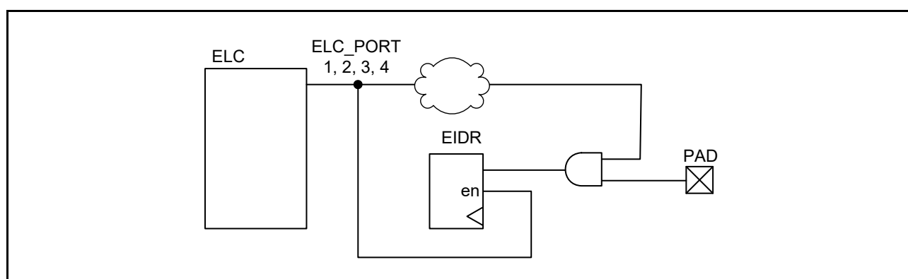
図 20.2 イベントポート入力データ
