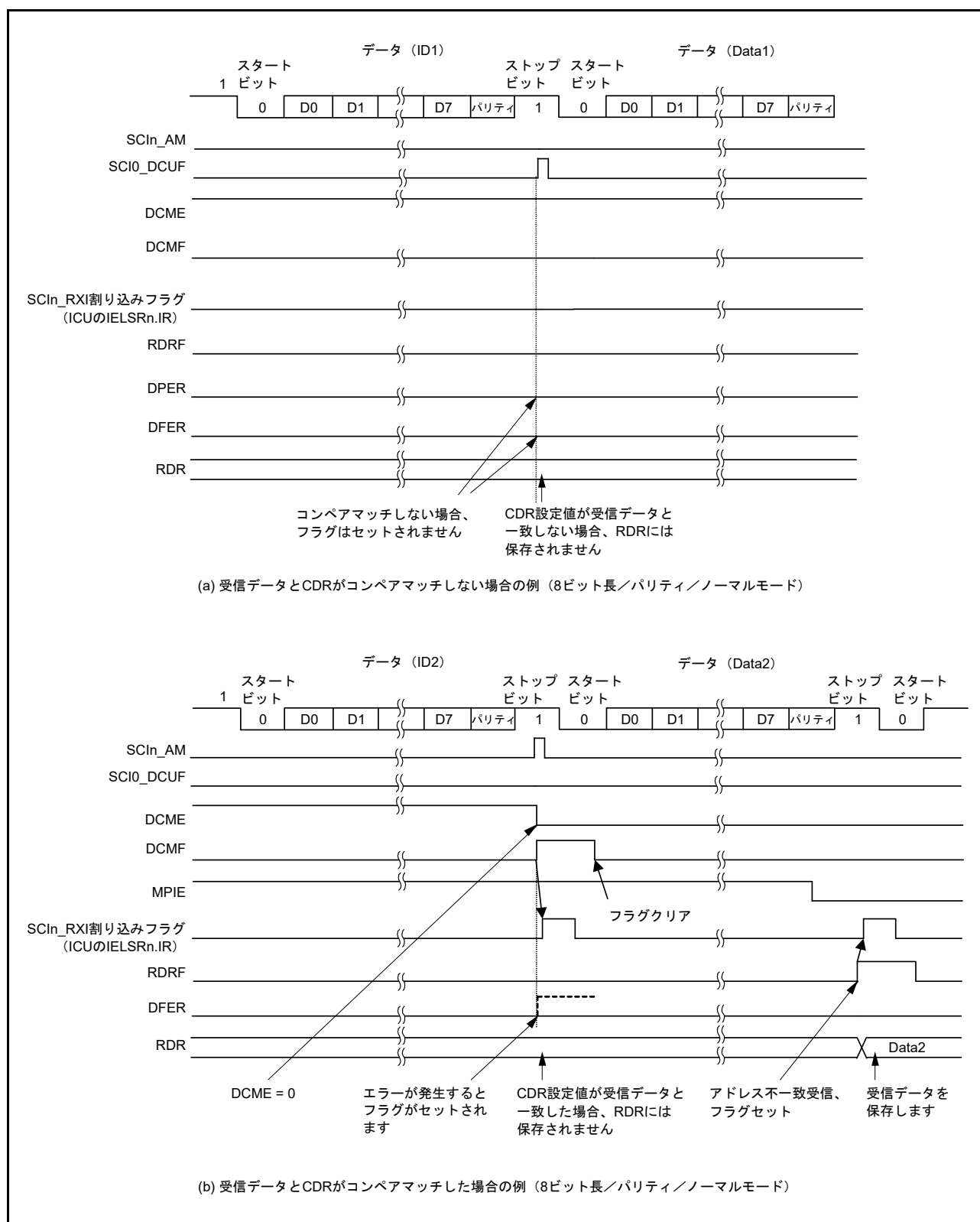
図 29.5 アドレス一致検出の例 (1) (通常モード)
