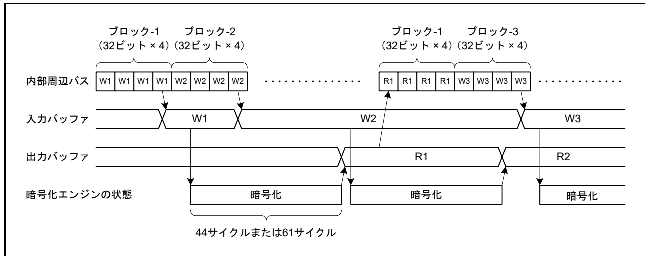
図 45.3 暗号化と復号タイミング (AES)
