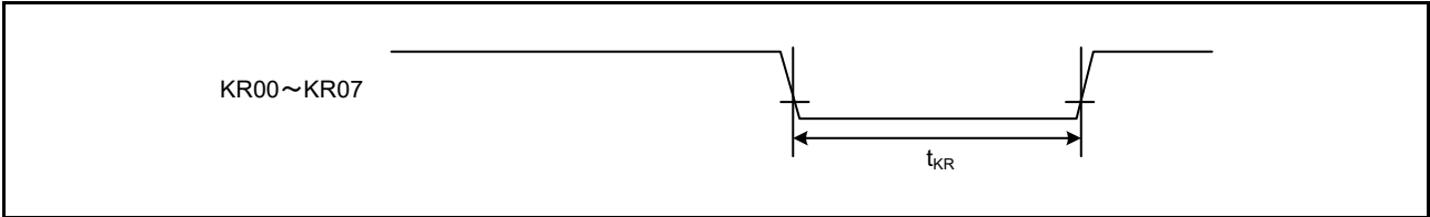
図 48.40 キー割り込み入力タイミング
