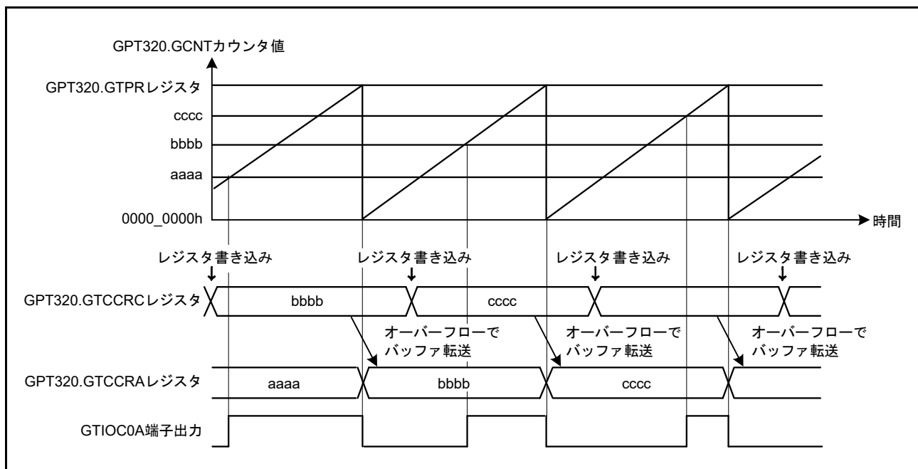
図 23.22 GTCRA、GTCCRB レジスタのバッファ動作例（アウトプットコンペア、アップカウント時ののこぎり波、GTCCRA レジスタのコンペアマッチで High 出力、周期の終わりで Low 出力の場合）
