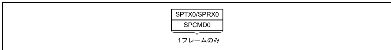
図 32.41 シーケンス動作時の SPI コマンドレジスタと送受信バッファの関係 (SPI1)
