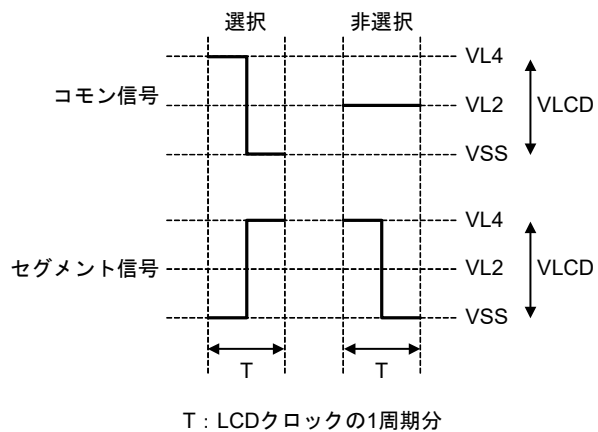
(b) 1/2バイアス法 (A波形)
