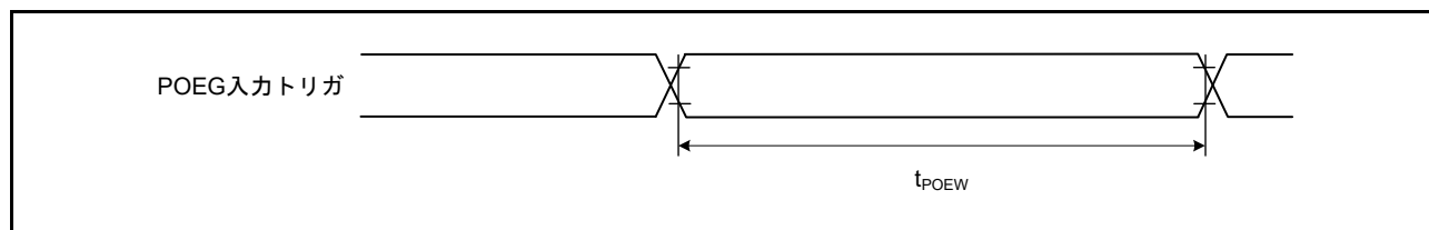
図 48.36 POEG 入力トリガタイミング
