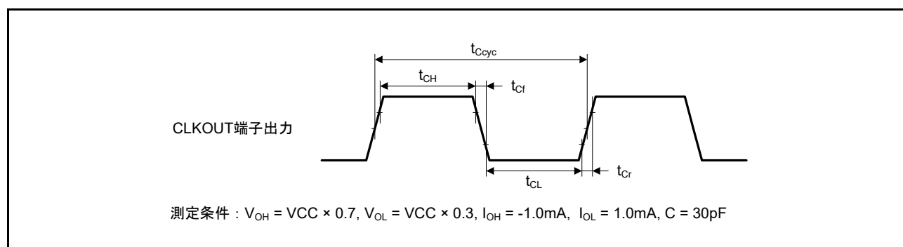
図 48.57 CLKOUT 出力タイミング
