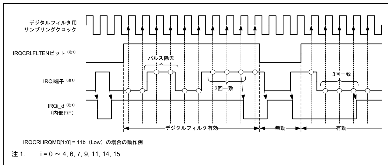
図 14.4 デジタルフィルタの動作例
