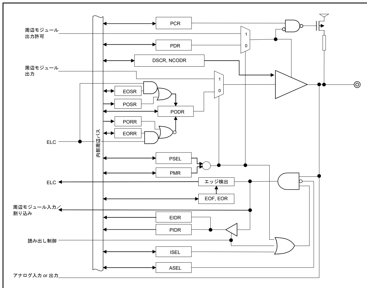
図 20.1 I/Oポートレジスタの接続図
