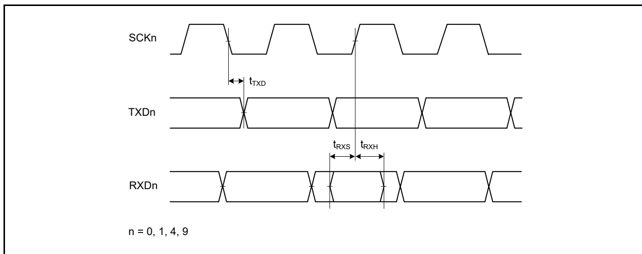
図 48.42 クロック同期式モードにおける SCI 入出力タイミング
