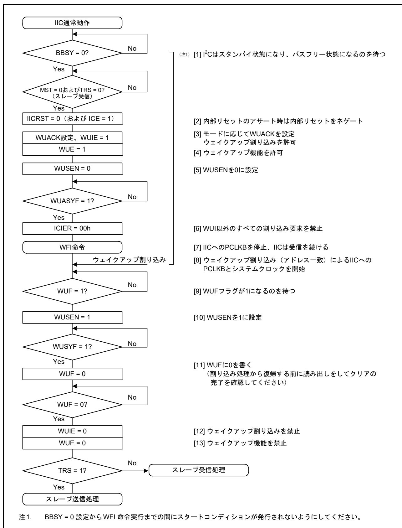
図 30.33 ノーマルウェイクアップモード2の動作例（スレープアドレス一致時のウェイクアップ割り込みによるウェイクアップの場合）
