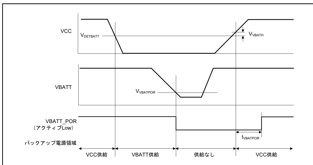
図 48.72 VBATT_POR リセットタイミング
