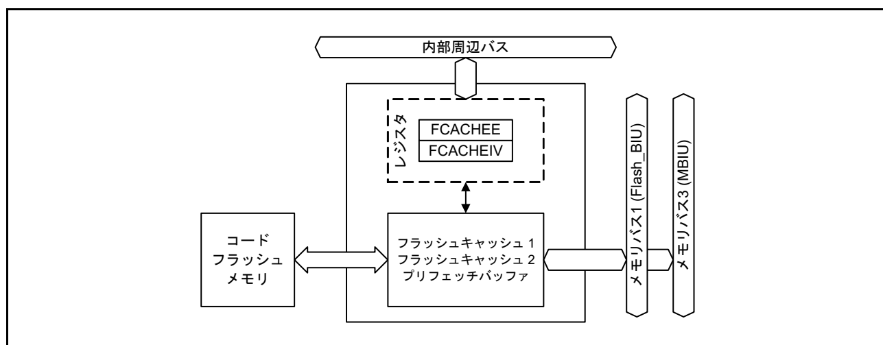
図 43.4 FCACHE のブロック図
