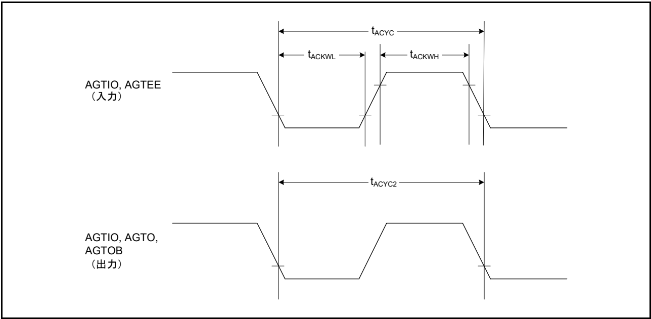
図 48.38 AGT 入出力タイミング
