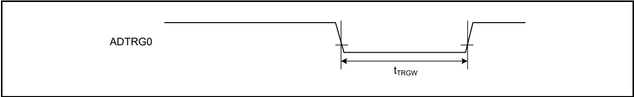
図 48.39 ADC14 トリガ入力タイミング
