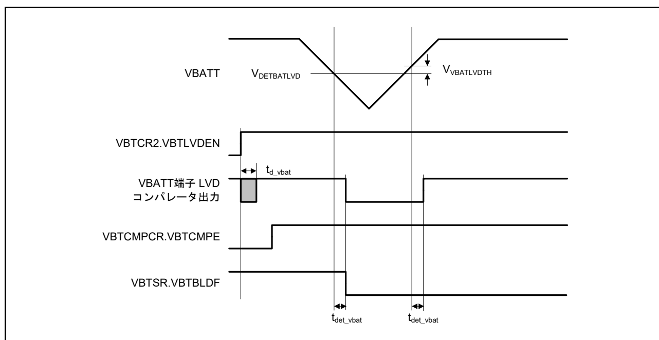
図 48.73 VBATT 端子電圧検出回路タイミング
