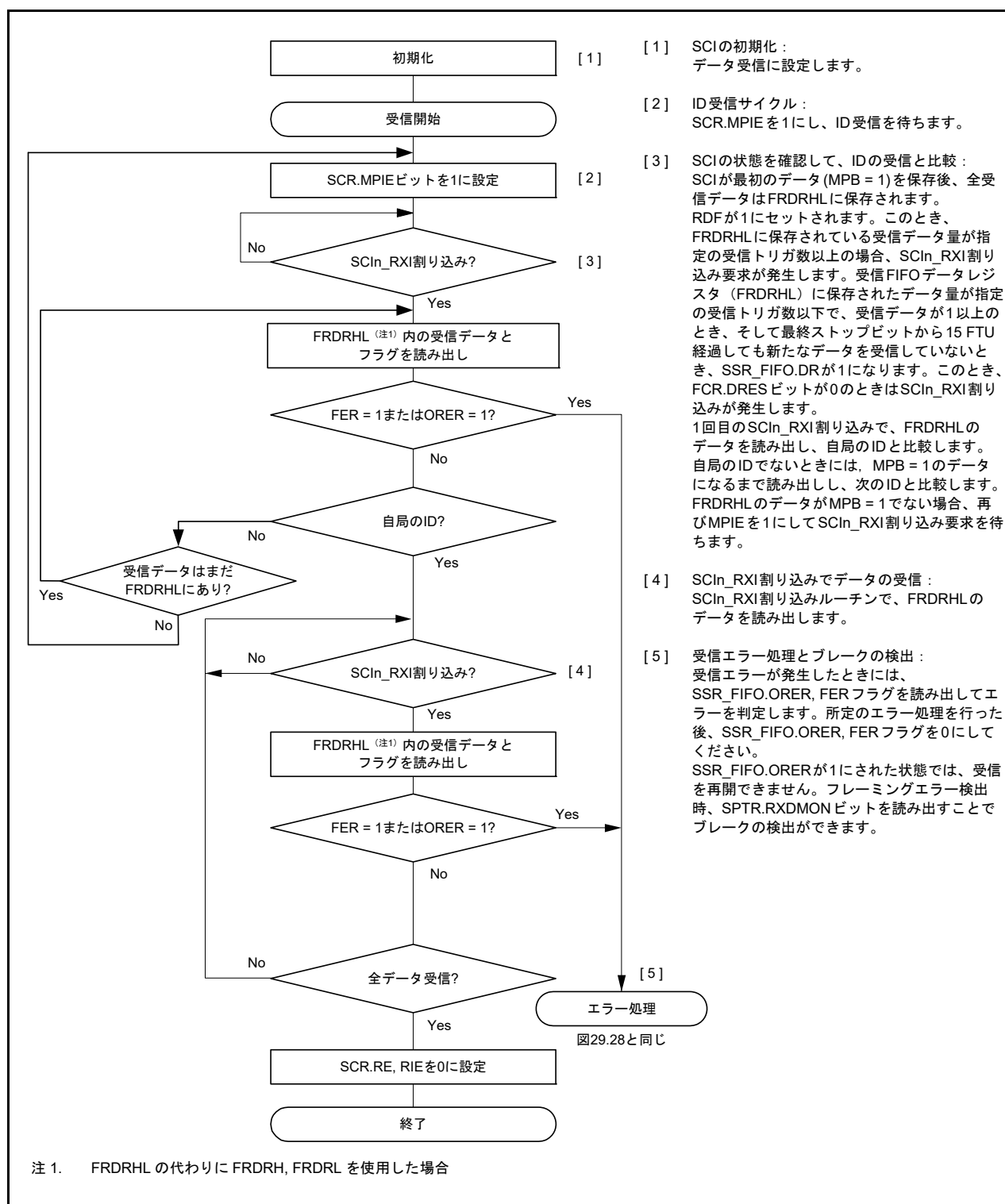
図 29.30 マルチプロセッサモードにおけるシリアル受信のフローチャート例 (FIFO 選択時)
