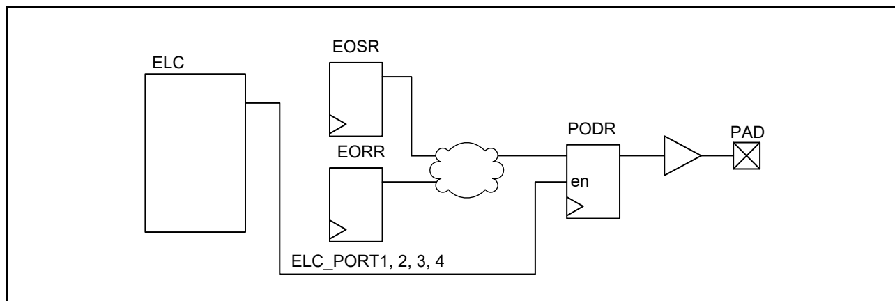
図 20.3 イベントポート出力データ
