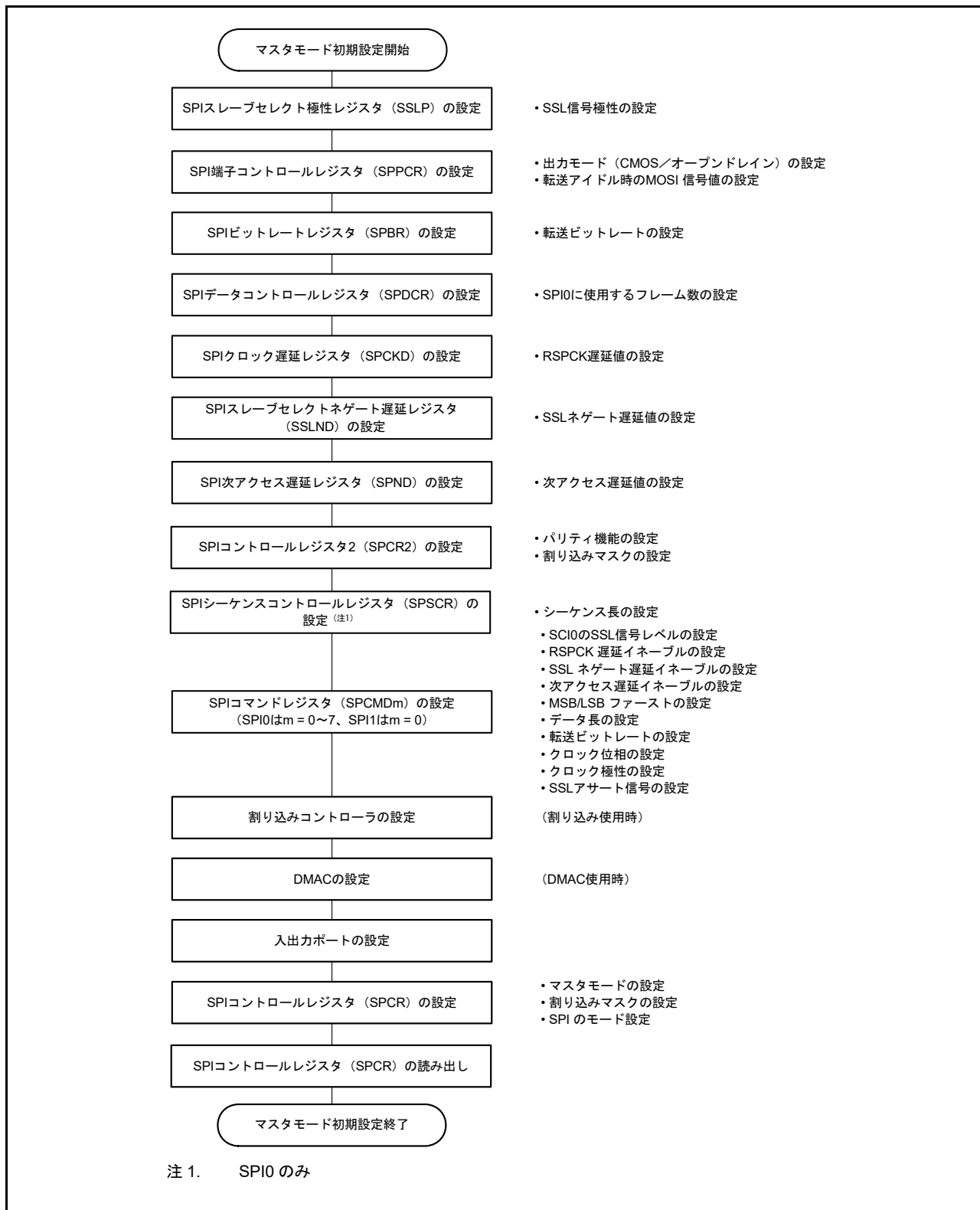
図 32.43 マスターモード時の SPI 動作の初期化フロー例
