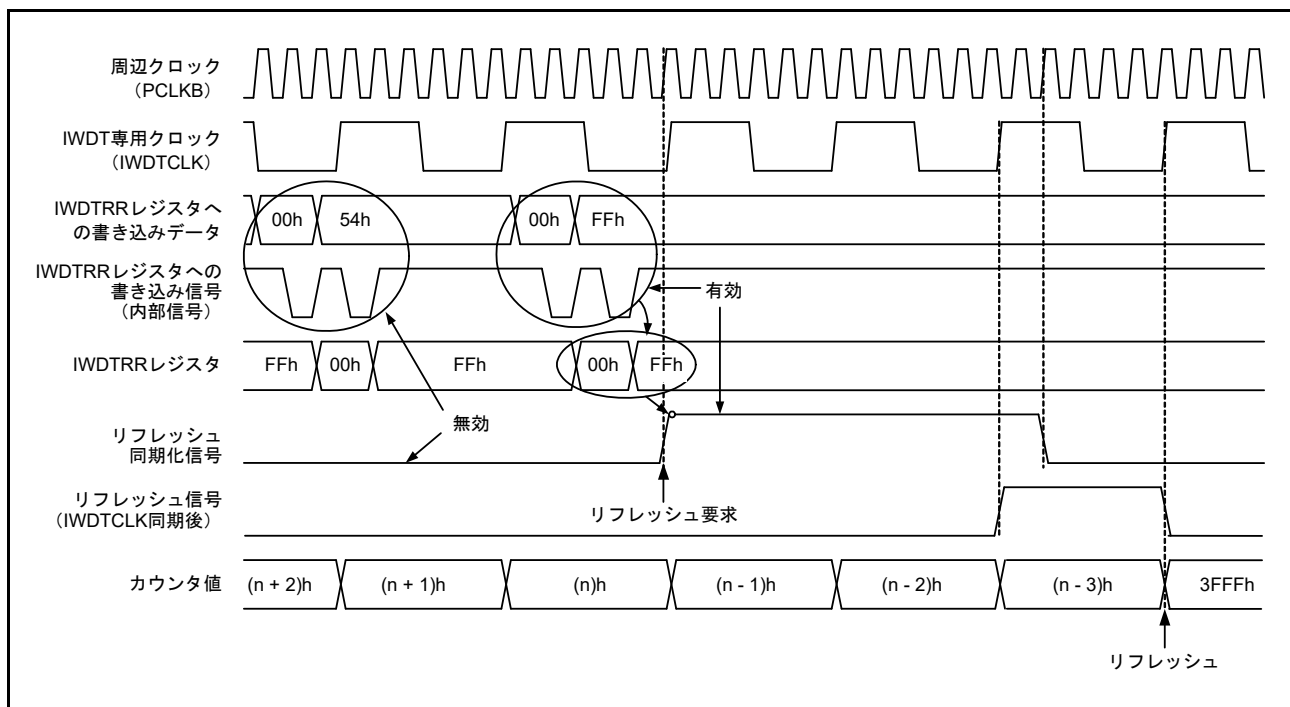
図 27.4 IWDT リフレッシュ動作波形 (OFS0.IWDTCCKS[3:0] = 0000b、OFS0.IWDTTOPS[1:0] = 11b の場合)
