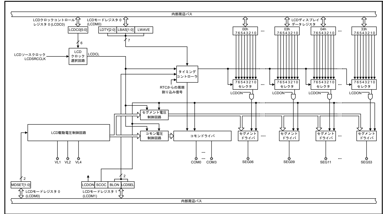
図 44.1 SLCDC のブロック図
