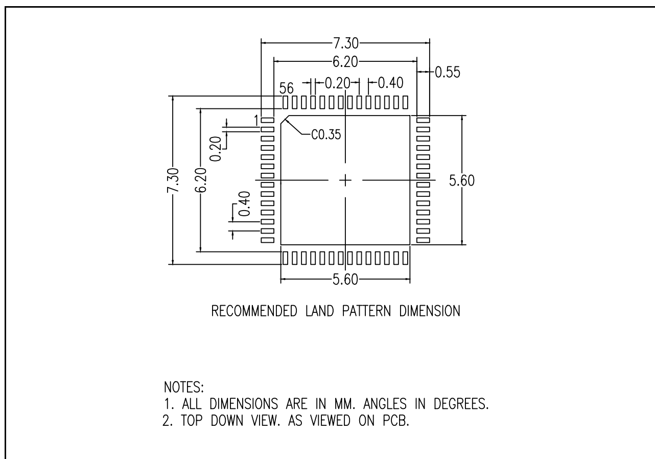
図 2.2 ランドパタン
