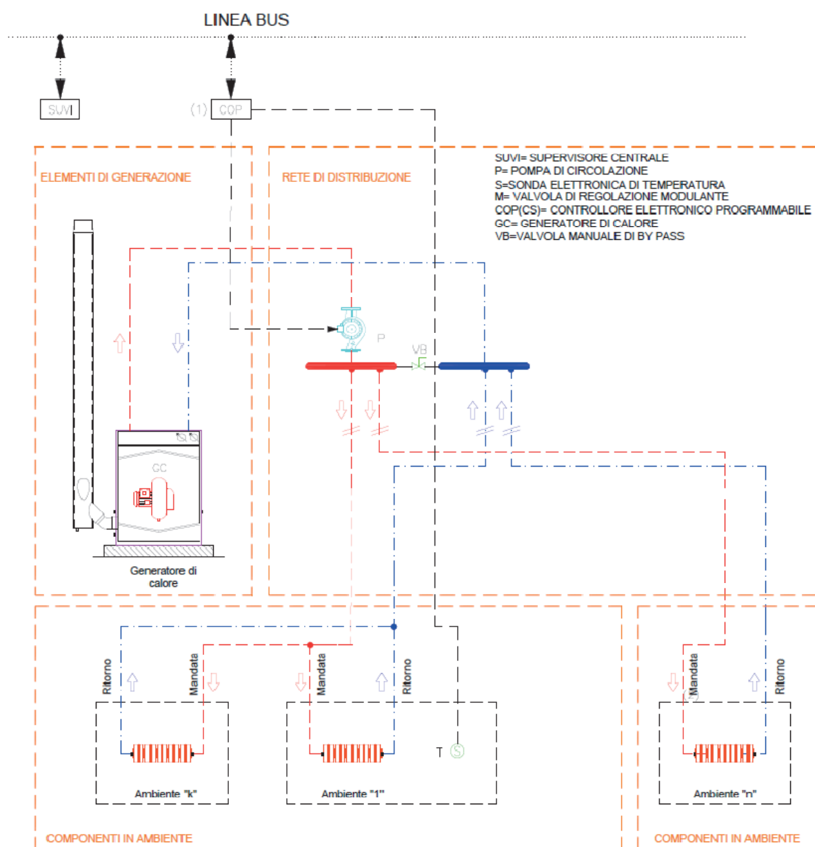
SCHEMA DI PRINCIPIO SE128
