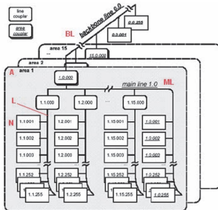
Figura 27 - Struttura di un sistema KNX
