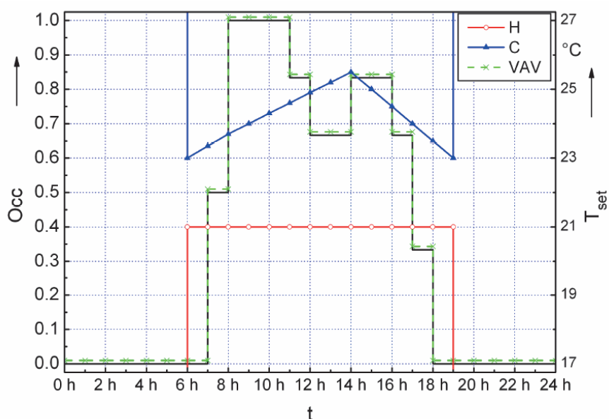
Figura 11 - Profili di riscaldamento / raffrescamento in classe A (caso uffici)
