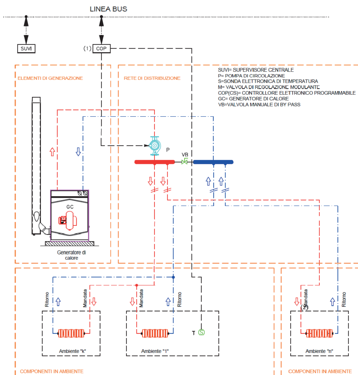
SCHEMA DI PRINCIPIO SE13A
