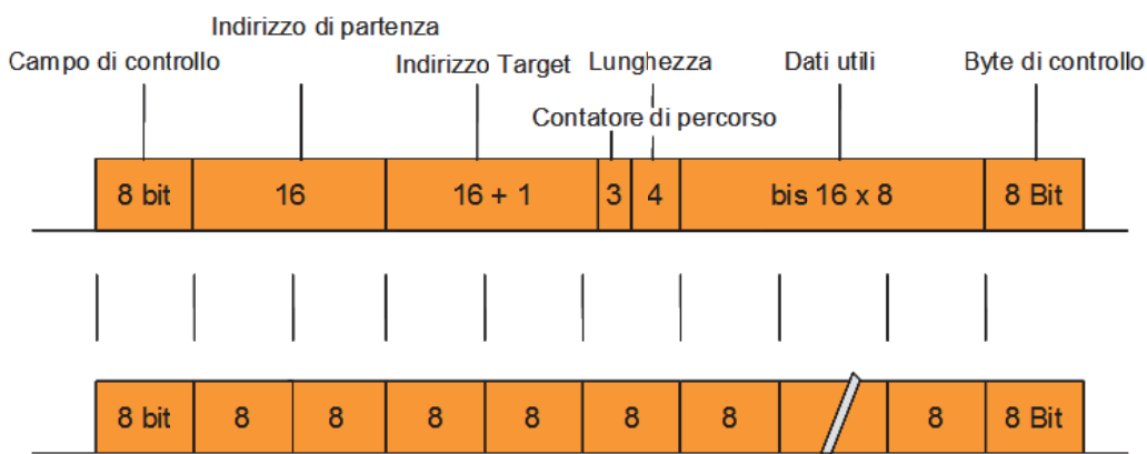
Figura 29 - Struttura del telegramma
