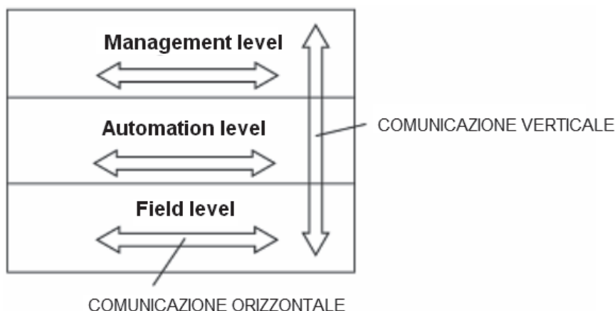
Figura 24 – Livelli di un sistema di automazione edifici
