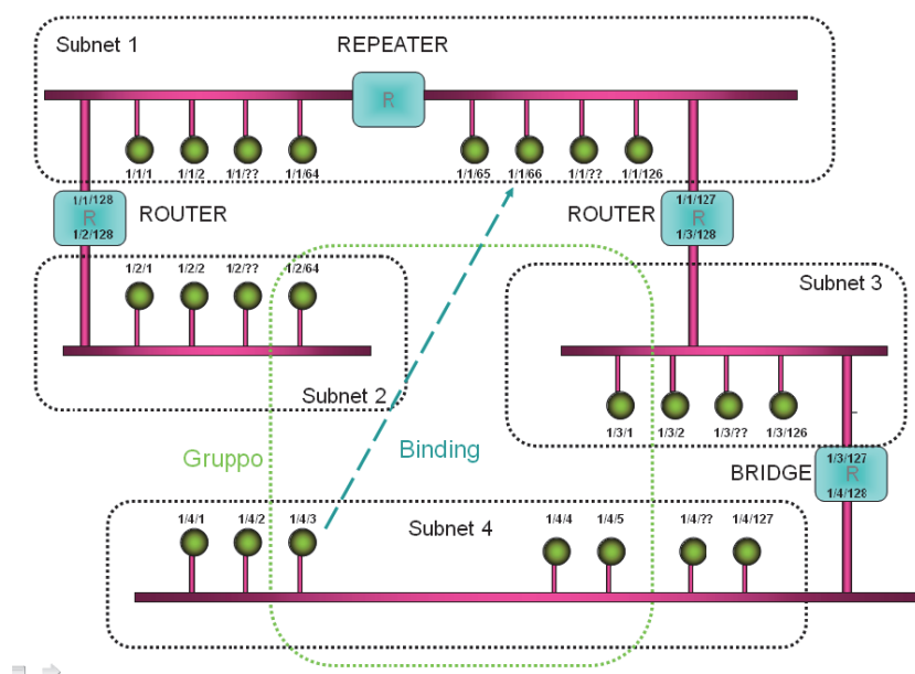
Figura 32 – Struttura Domain / Subnet / Node
