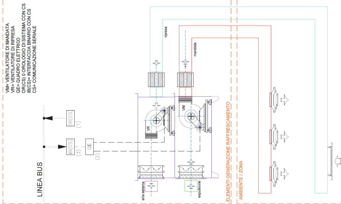
SCHEMA DI PRINCIPIO SE54BC
