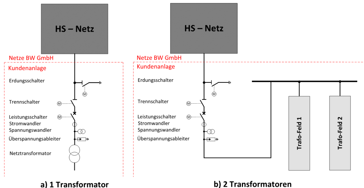
Abbildung 2: Aufbau Hochspannungsanschluss
