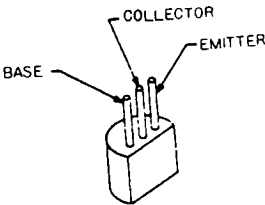
2SA564A
