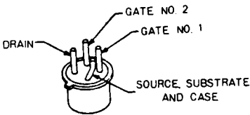
3SK51-03
