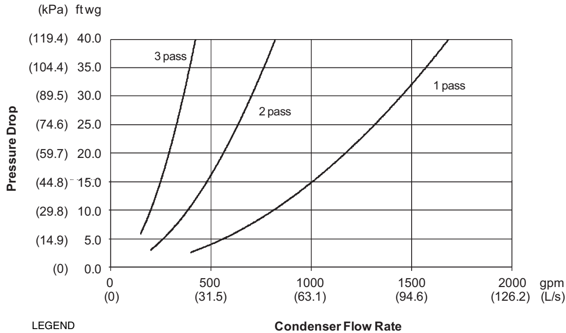
30XW150-200 CONDENSER NIH FLANGE
