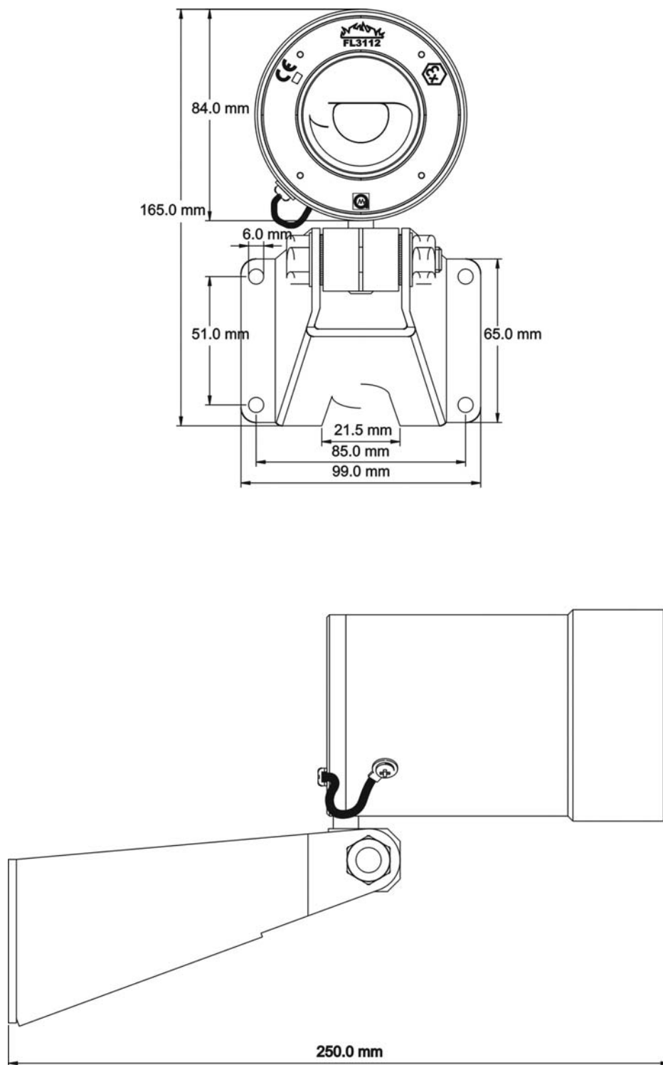
Figure 3-B Schéma d'encombrement
