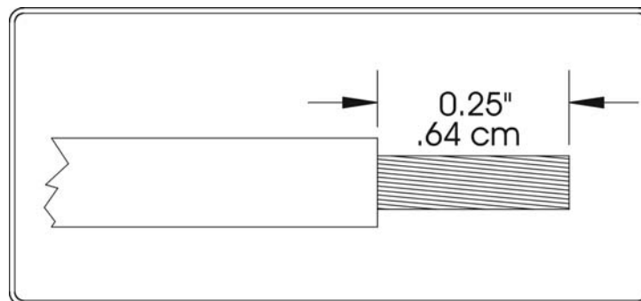
Figure 3-D Longueur de dénudation
