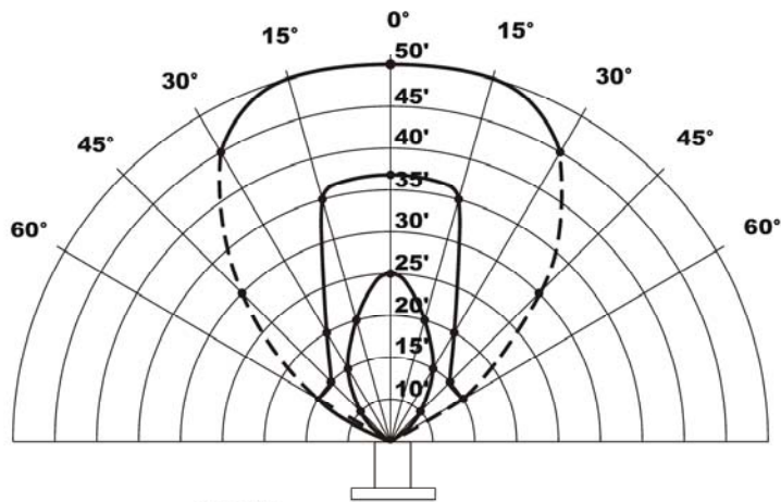
Figure 3-A FL3112 Champ de visibilité
