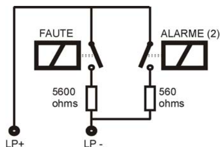
Figure 3-F Sorties boucle de champ
