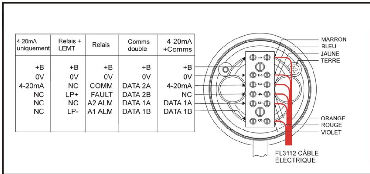
Figure 3-C Socle d'assemblage avec bloc de dérivation
