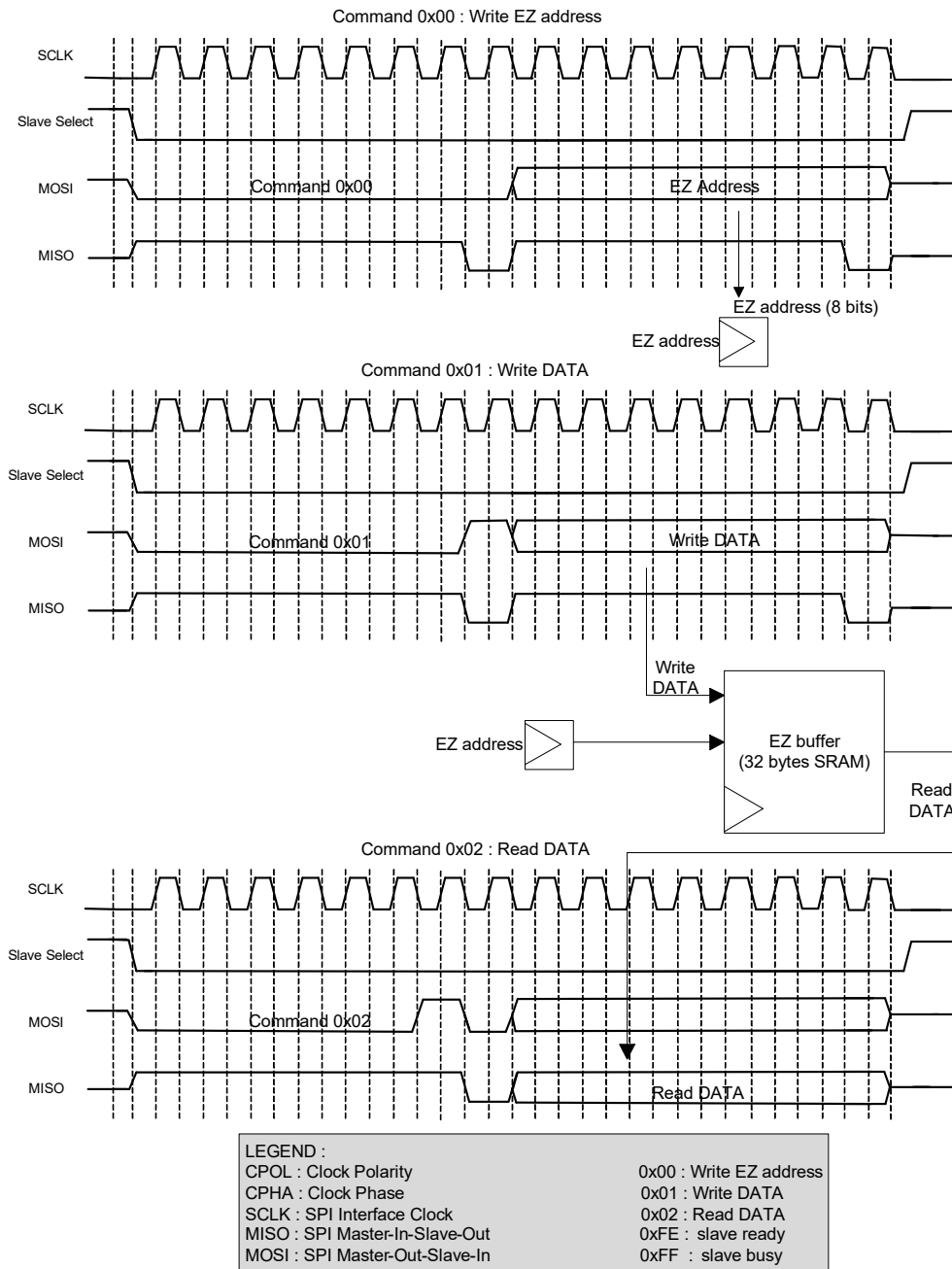
Figure 14-7. EZSPI Example
