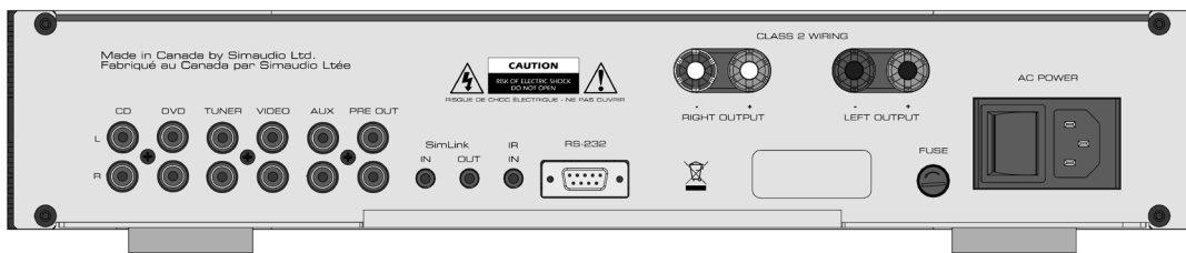
Figure 2: Panneau arrière 250i
