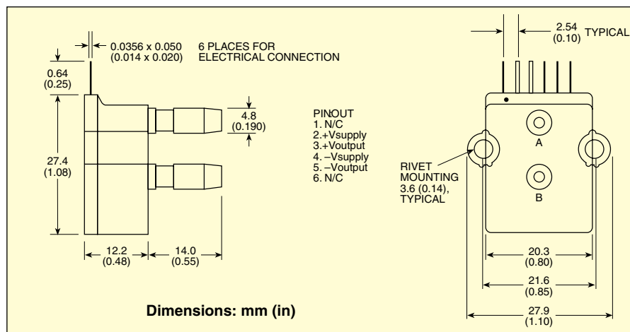
Actual size.
