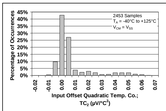
FIGURE 2-3: Input Offset Quadratic Temp. Co.
