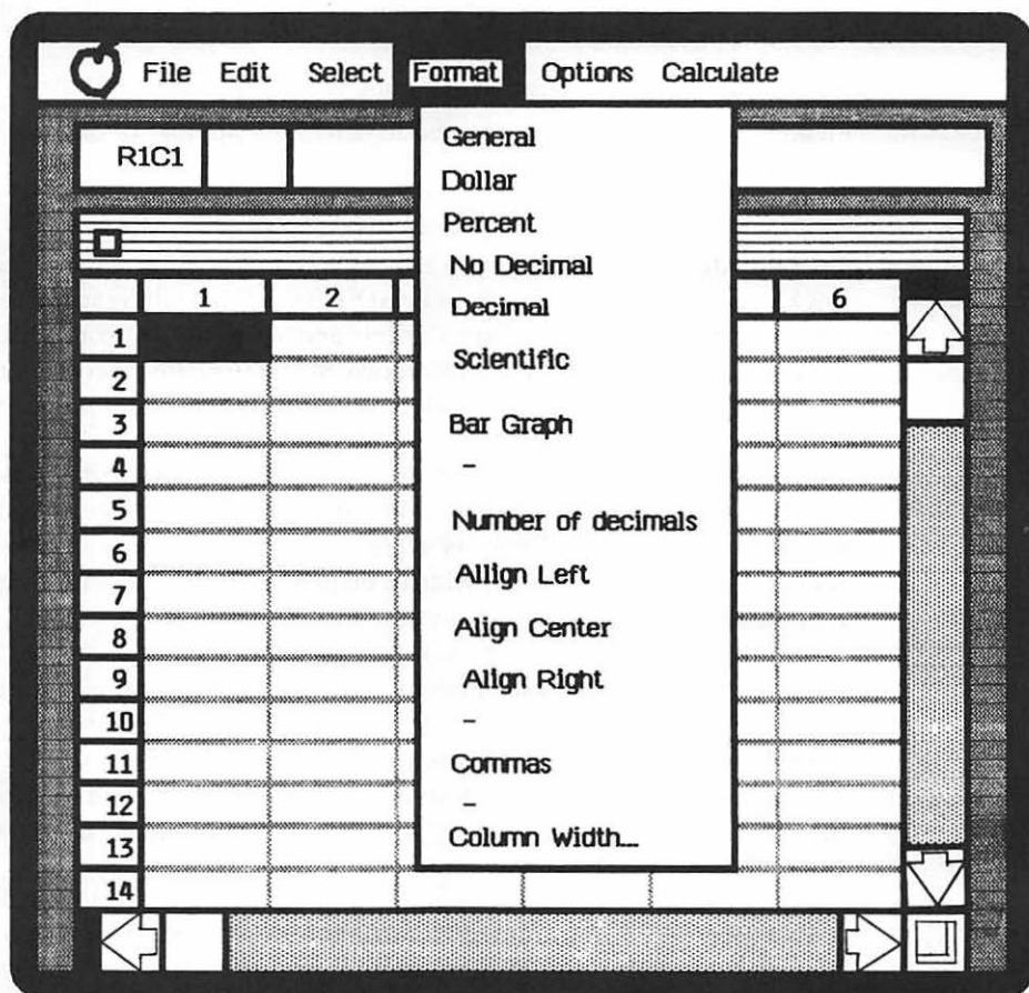
Figure 2.4 Format Menu.
