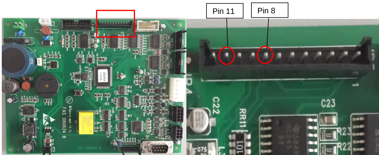
Hauptplatine
