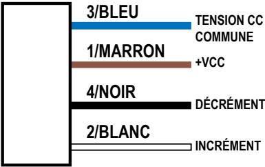
Illustration 33. Schéma de câblage pour l'incrémentation/la décrémentation du compteur
