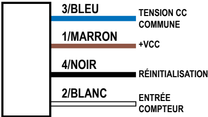
Illustration 32. Schéma de câblage pour l'entrée du compteur
