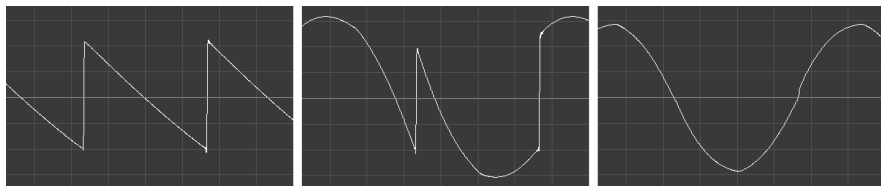
Niveau du suboscillateur = 0 % Niveau du suboscillateur = 50 % Niveau du suboscillateur = 100 %
