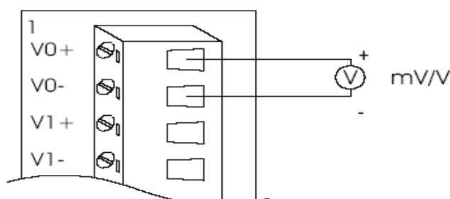
Figure 1.5 Millivolt and Volt Input
