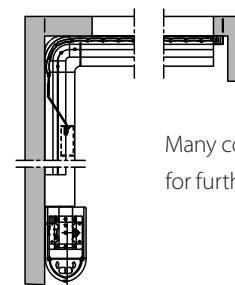
SeceuroGlide Vertico: White Colour Finish
