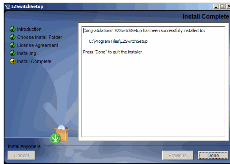
FIGURE 3 EZSwitchSetup Installer
