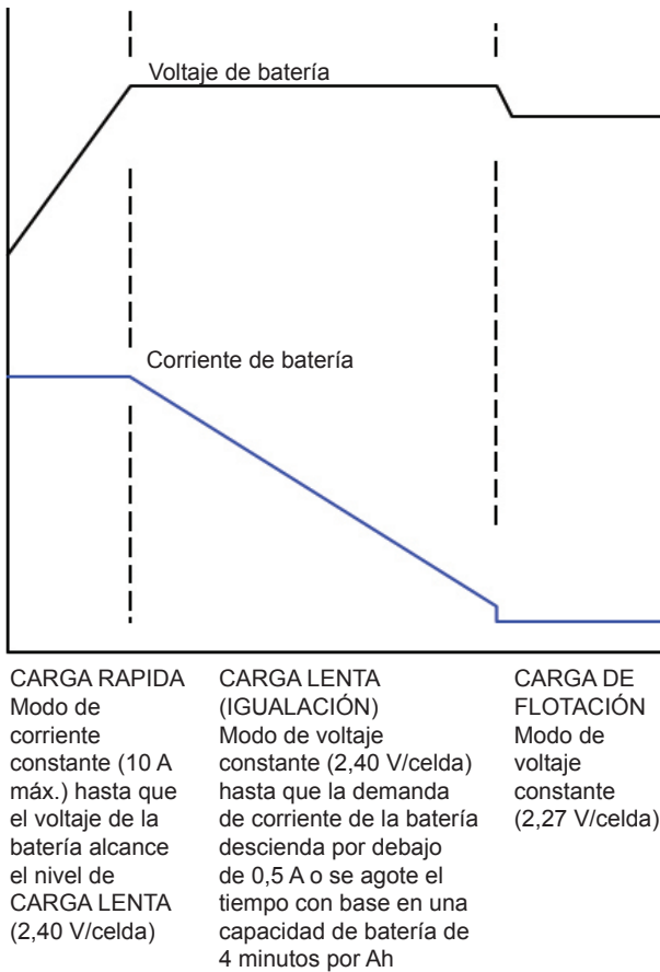
Fig. 1-2, Modos de cargador de 3 etapas
