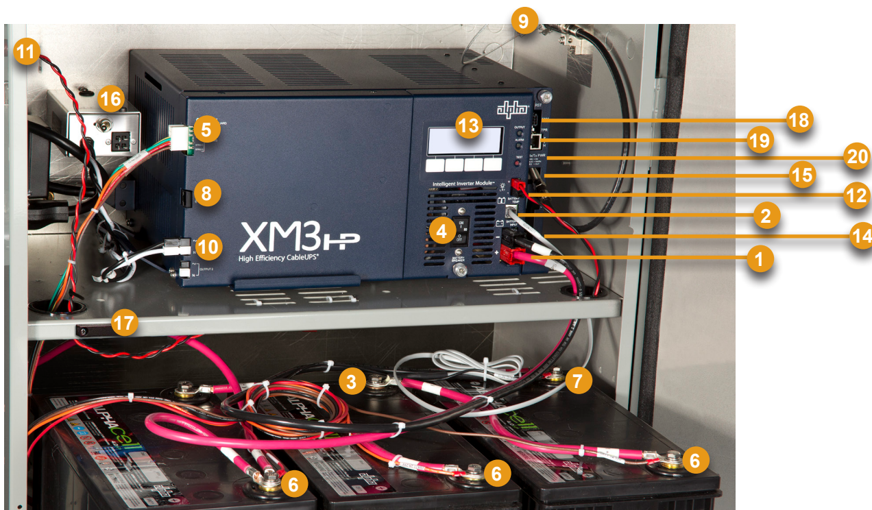
Fig. 2-4, Instalación del XM3-HP
