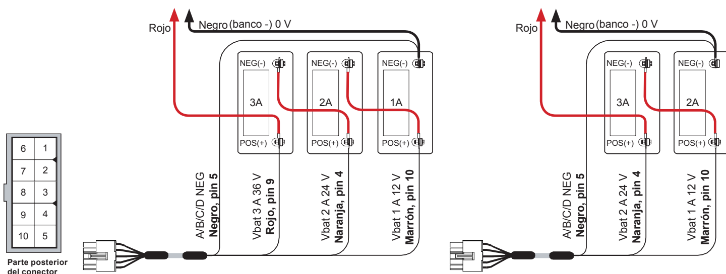
Fig. 1-10, Diagrama de cableado de banco de batería único (con arnés del SAG integrado ilustrado)
