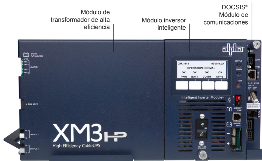
Fig. 1-5, Panel frontal, fuente de potencia XM3-HP
