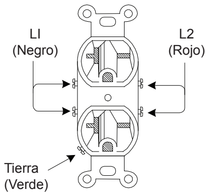
Cableado típico de receptáculo de 240 V CA 20 A, 6-20 R (N/P 531-008-19)
