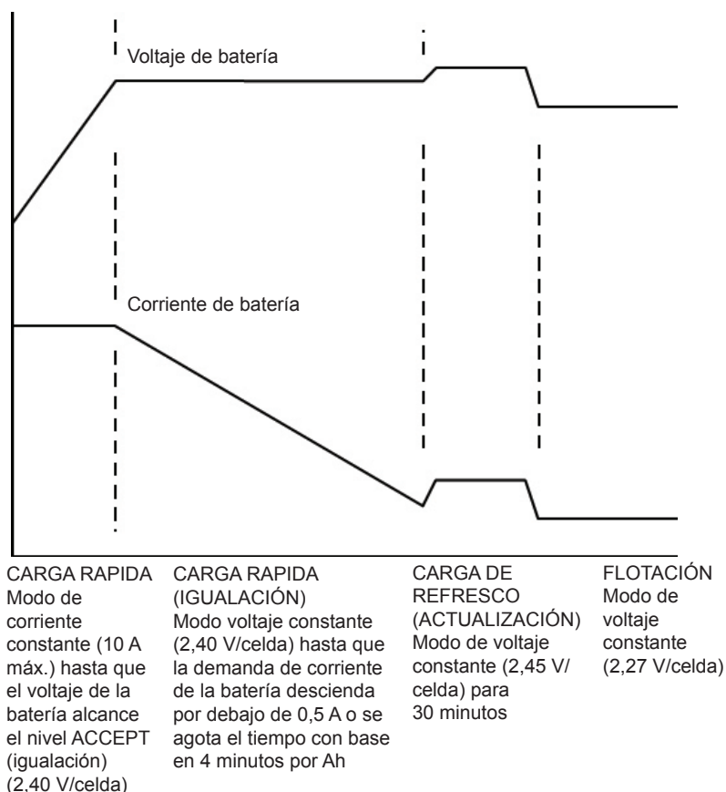
Fig. 1-3, Modos de cargador de 4 etapas
