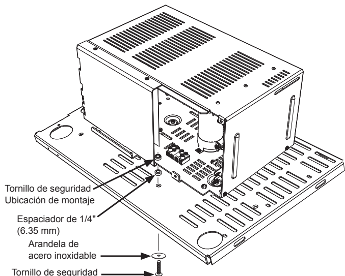
Figura 2-3, Instalación del tornillo de seguridad
