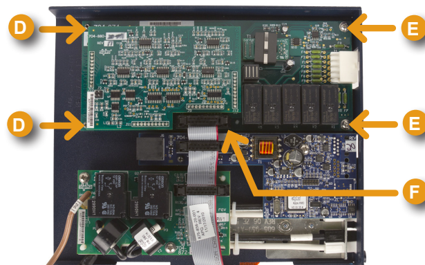
Fig. 2-17, Ubicaciones del cable plano, los tornillos y el soporte de la tarjeta SAG
