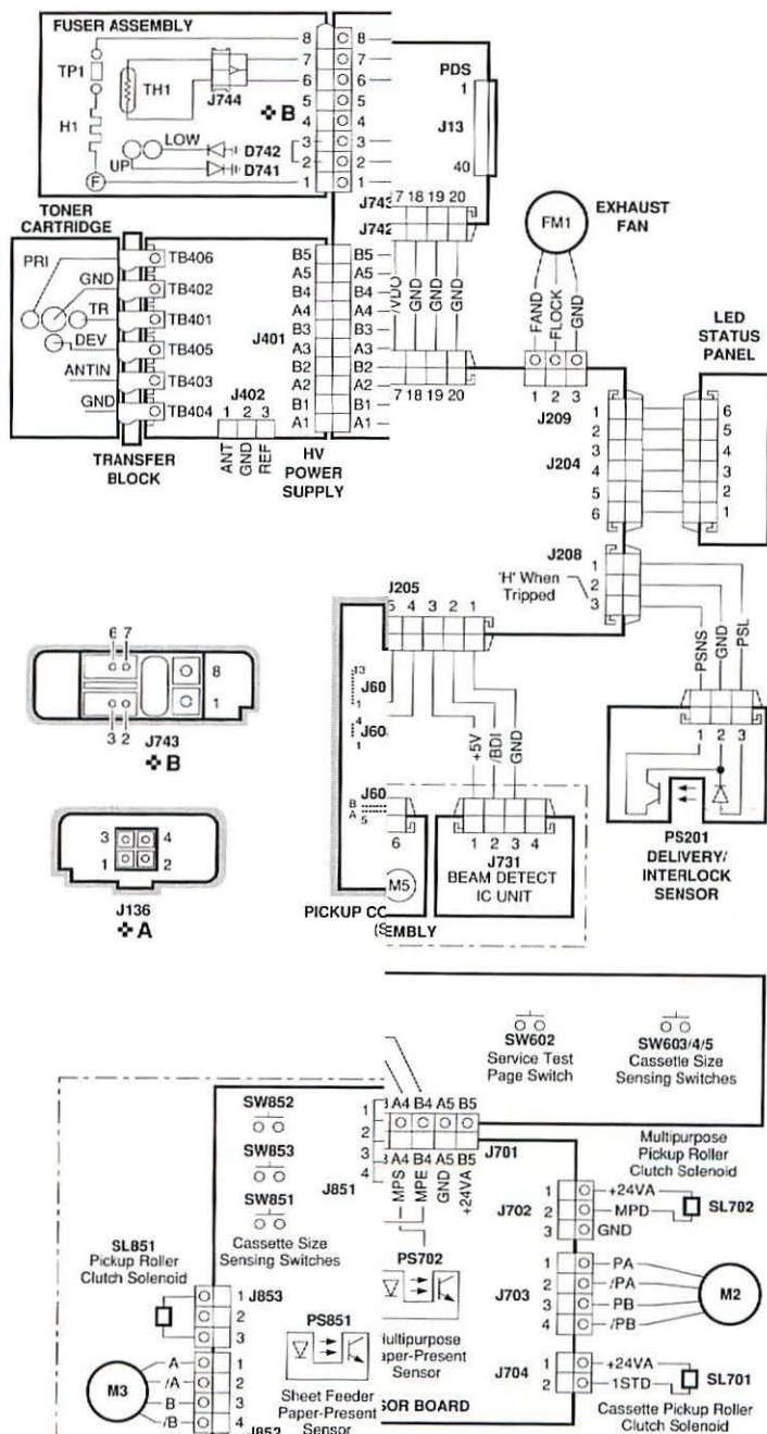
LaserWriter Pro 600/630 Wiring Diagram
