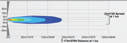
XIL-200 | 4006317 - EURO BEAM
