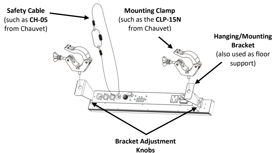
COLORstrip Mini Mounting Diagram
