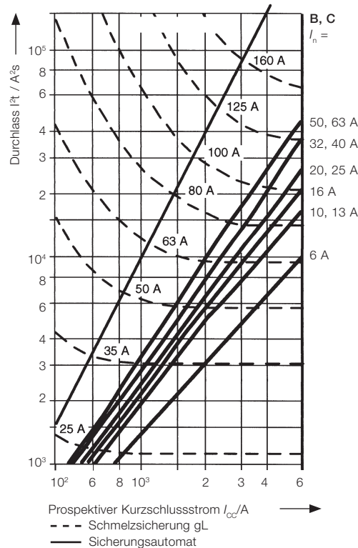
Abb. 2 Durchlassenergie I^2t
