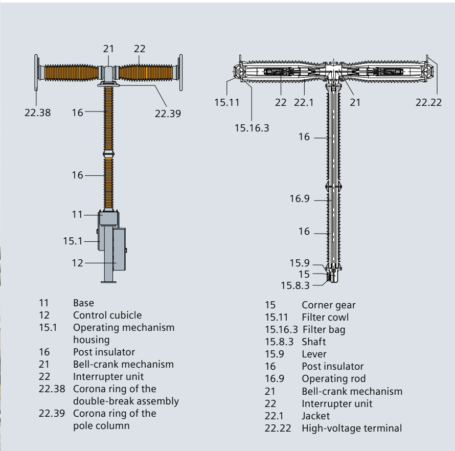
Fig. 6: 3AP2 FI 550 kV pole
