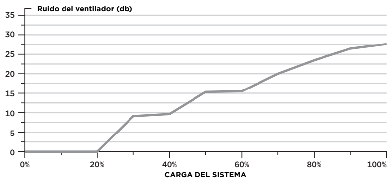
Curva de ruido del ventilador de la fuente de alimentación Corsair SF450
