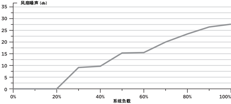
Corsair SF450 电源风扇噪声曲线
