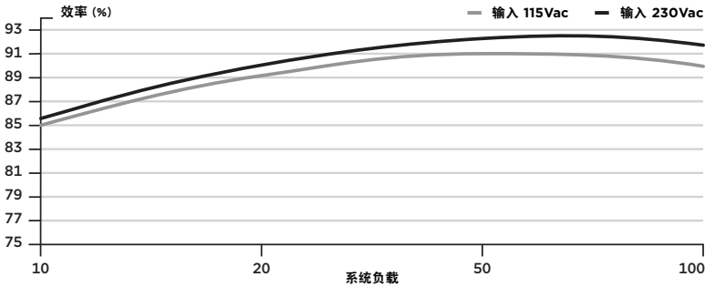
Corsair SF450 电源效率
