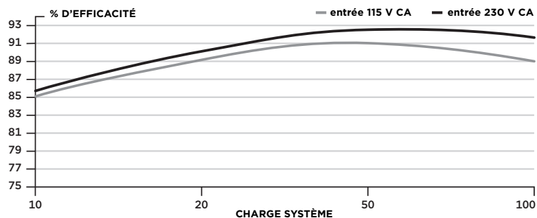
Efficacité de l'alimentation Corsair SF600
