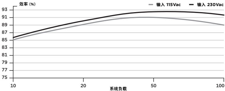
Corsair SF600 电源效率
