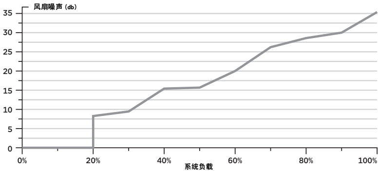
Corsair SF600 电源风扇噪声曲线
