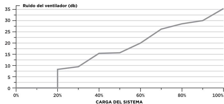
Curva de ruido del ventilador de la fuente de alimentación Corsair SF600
