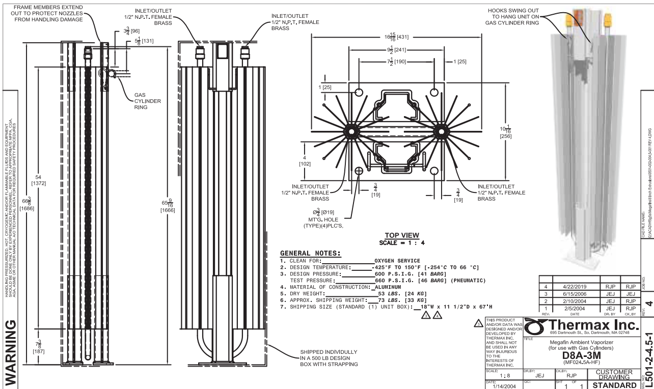
D8A-3M Vaporizer
