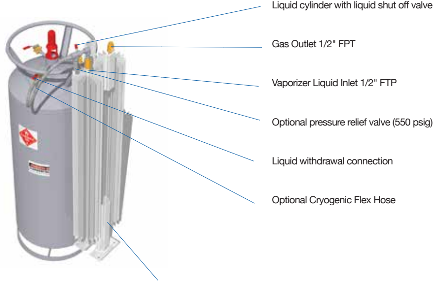
D8A-3M Vaporizer
