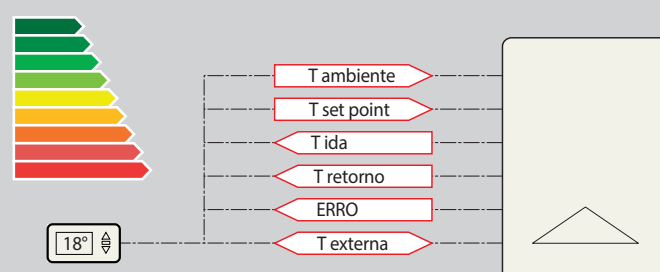
Fig. 25: Termostatização com protocolo de comunicação avançado
