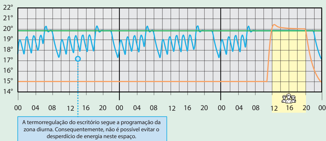
Fig. 23: Diferenças entre diversas soluções de termorregulação no caso de instalações autónomas de radiadores com duas zonas
