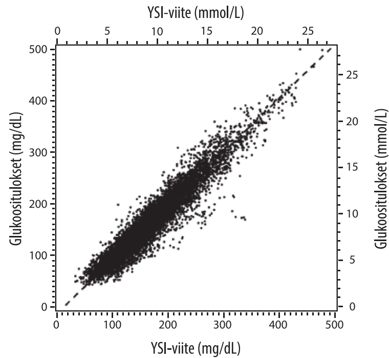
Taulukko 1. Sensorien regressioanalyysi verrattuna YSI-viitteen
