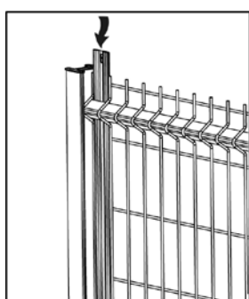
glissez la lame de rive gauche
