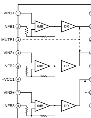
IC711 : LA7104M Double Scart Interface
