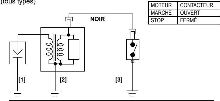
DÉMARREUR ÉLECTRIQUE (à frein de volant)
