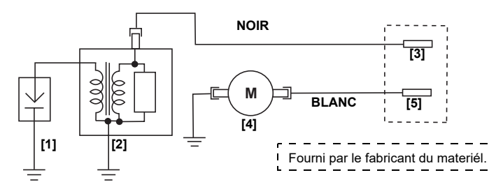
DÉMARREUR ÉLECTRIQUE (à frein-embayage)
