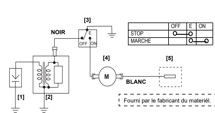
DÉMARREUR ÉLECTRIQUE (à frein-embayage)
