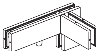
Sidelite Transom Fin Patch (PFT-41)
