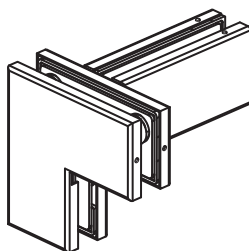
Sidelite Transom Fin Patch (PFT-61)
