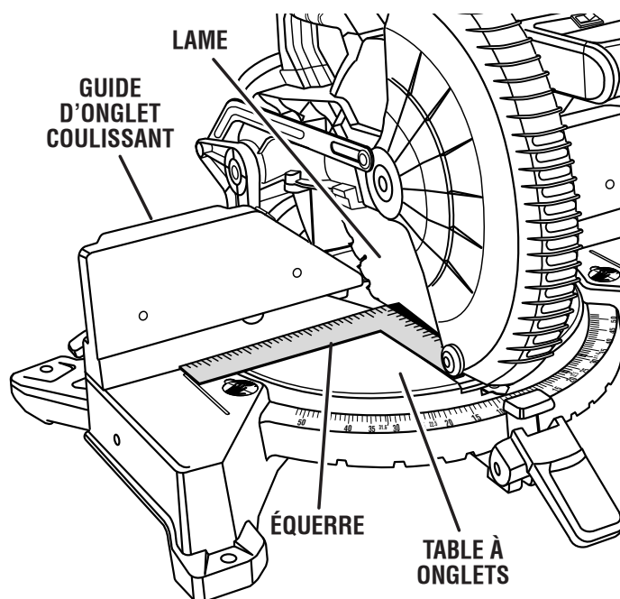
VUE DE LA LAME PAS D'ÉQUERRE AVEC LE GUIDE, DES RÉGLAGES SONT NÉCESSAIRES Fig. 20
