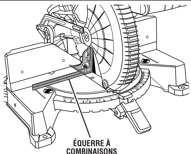
VUE DE LA LAME PAS D'ÉQUERRE AVEC TABLE À ONGLETS, DES RÉGLAGES SONT NÉCESSAIRES
