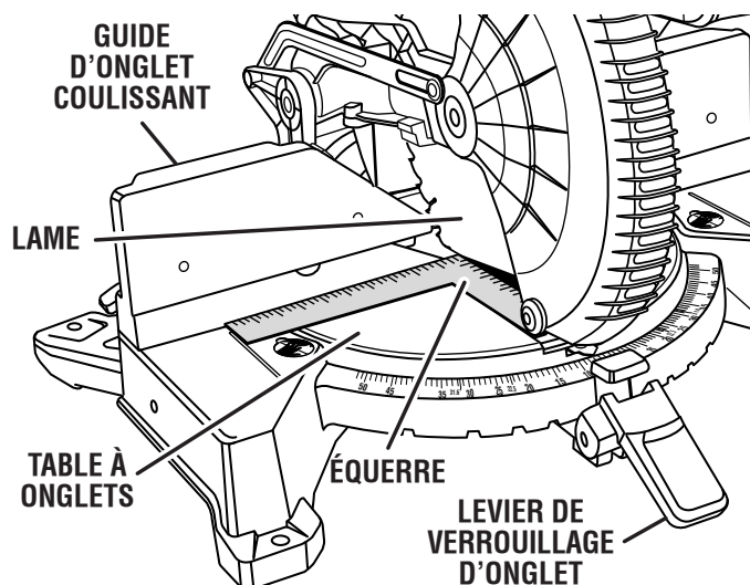
VUE DE LA LAME PAS D'ÉQUERRE AVEC LE GUIDE, DES RÉGLAGES SONT NÉCESSAIRES Fig. 19
