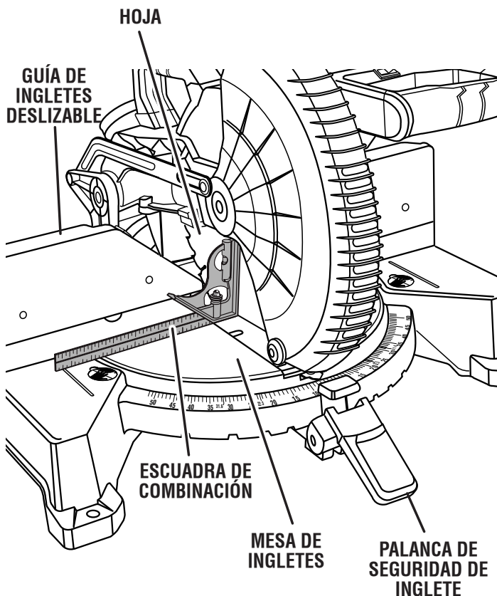
VISTA CORRECTA DE LA HOJA A ESCUADRA CON LA MESA DE INGLETES
