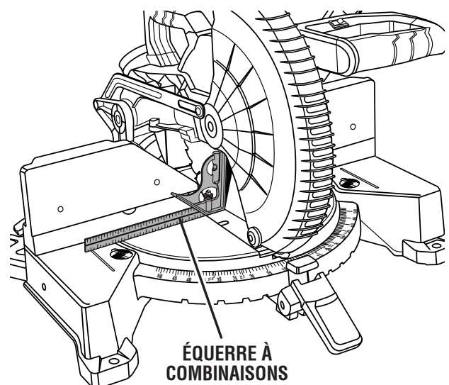
VUE DE LA LAME PAS D'ÉQUERRE AVEC LA TABLE, DES RÉGLAGES SONT NÉCESSAIRES
