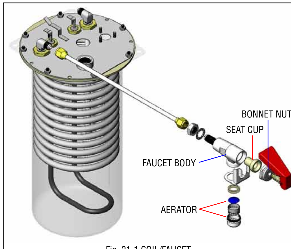
Fig. 21-1 COIL/FAUCET
