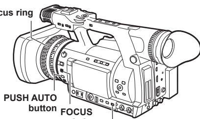
AUTO/MANUAL switch
