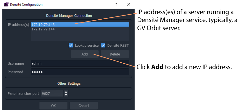
Fig. 2-41: iControl/Densité Configuration Dialog
