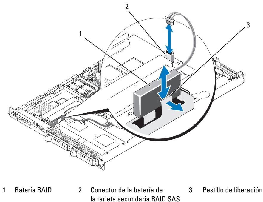
Figura 3-10. Instalación de la batería RAID SAS
