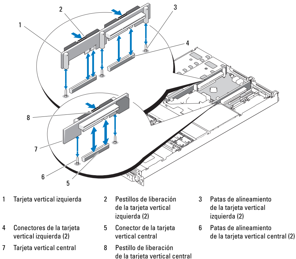
Figura 3-19. Extracción de la tarjeta vertical de expansión
