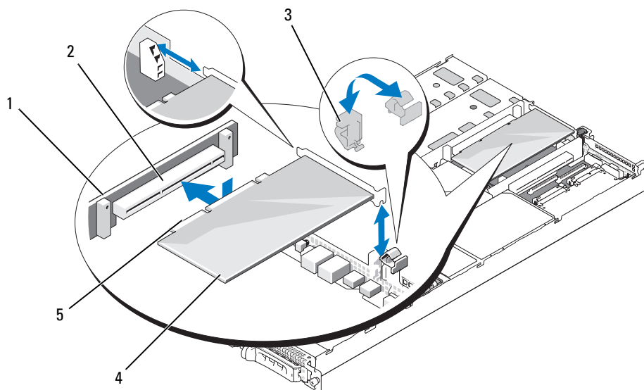
Figura 3-11. Instalación de una tarjeta de expansión
