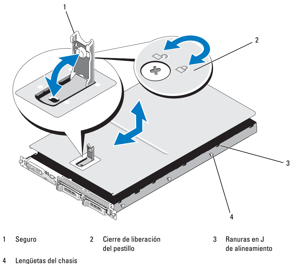
Figura 3-3. Extracción de la cubierta
