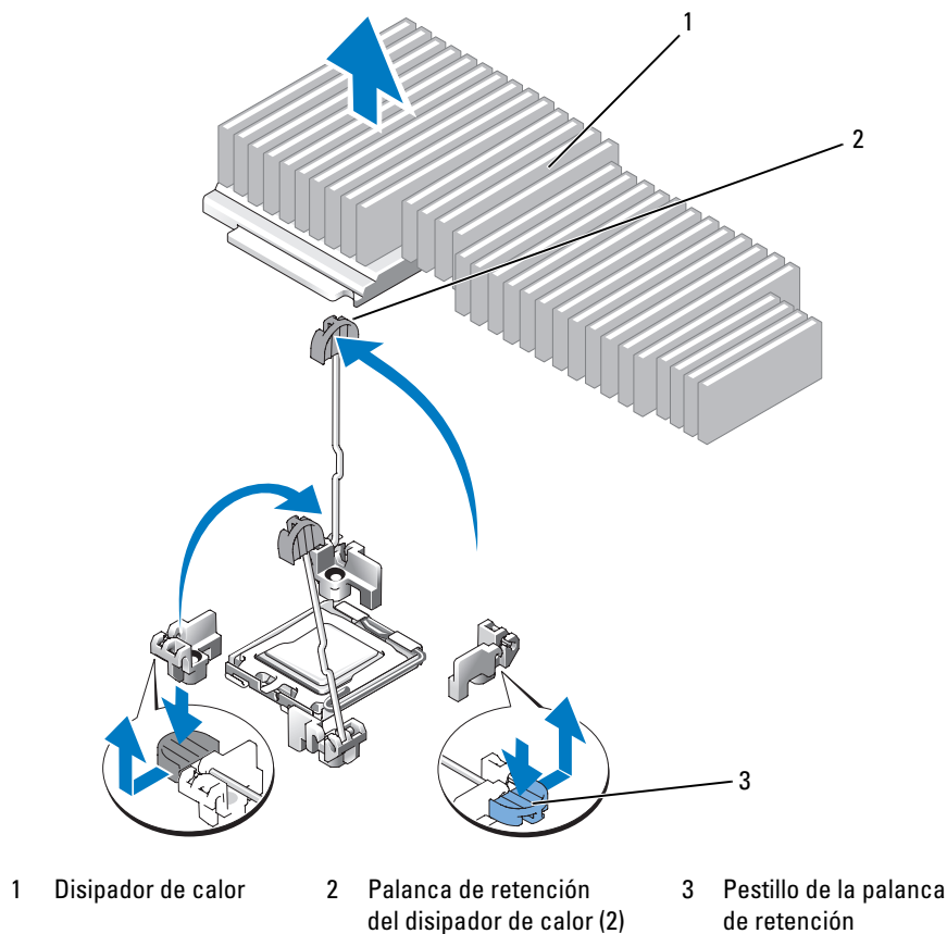
Figura 3-13. Instalación y extracción del disipador de calor
