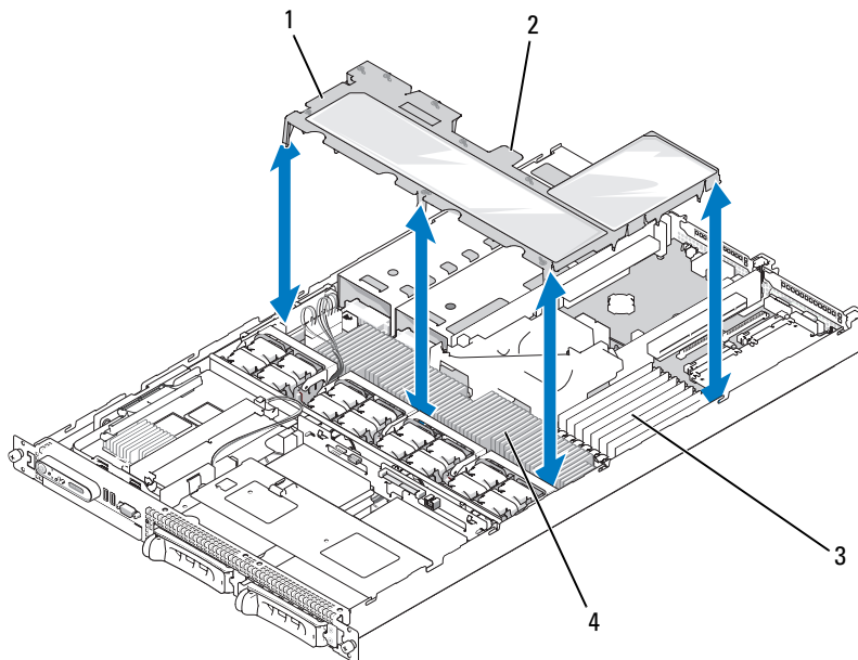
Figura 3-6. Cubierta de refrigeración de la memoria
