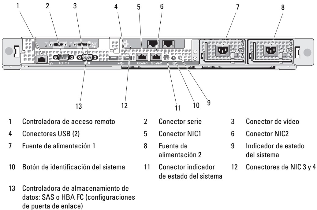
Figura 1-3. Componentes e indicadores del panel posterior
