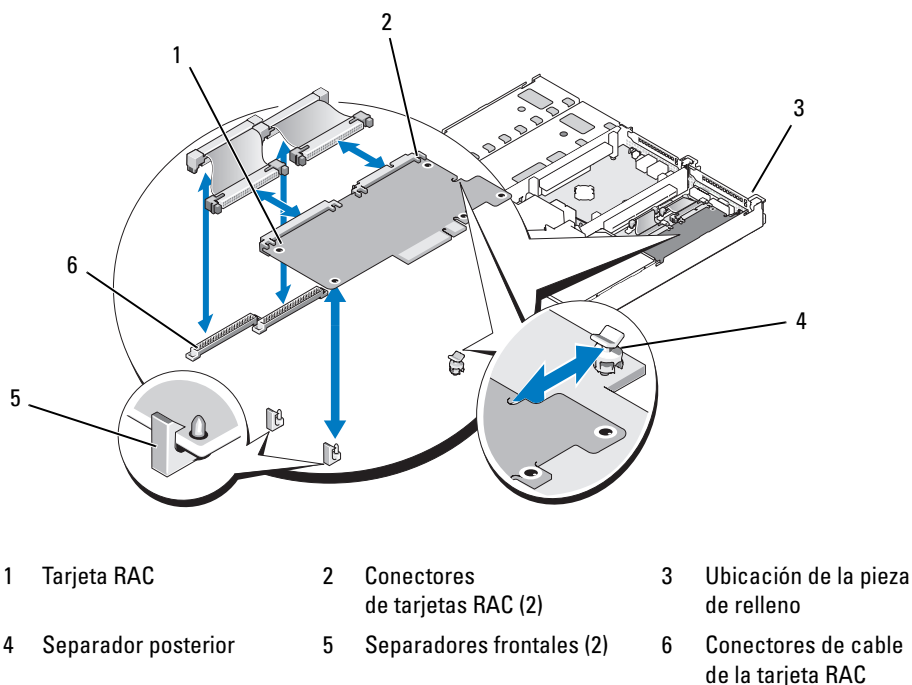
Figura 3-15. Instalación de una tarjeta RAC
