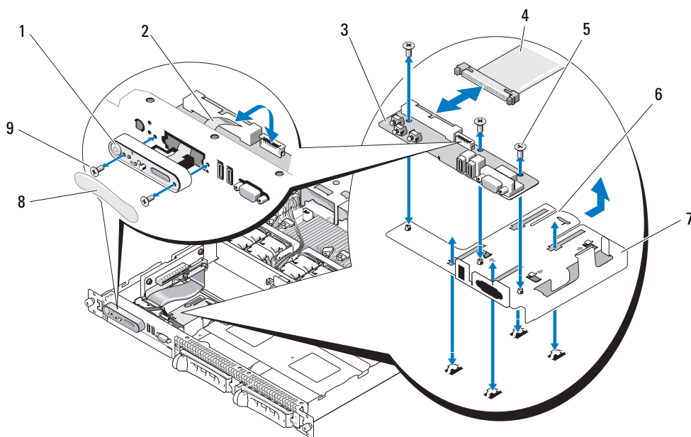
Figura 3-22. Instalación y extracción del panel de control
