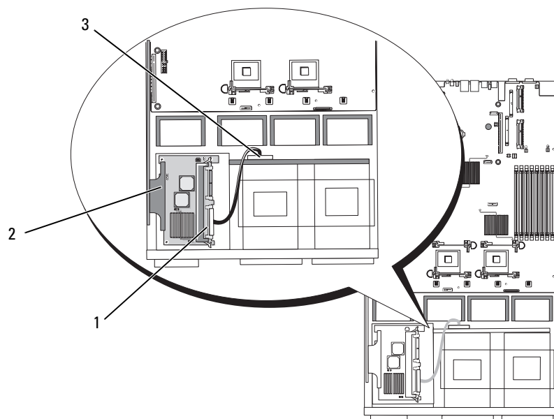
Figura 3-9. Colocación de los cables para la tarjeta controladora secundaria RAID SAS
