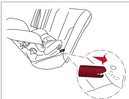
Voltado para trás com ganchos tipo rígido – etapa 2
