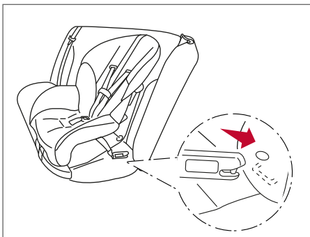
Voltado para frente tipo gancho rígido – etapa 2
