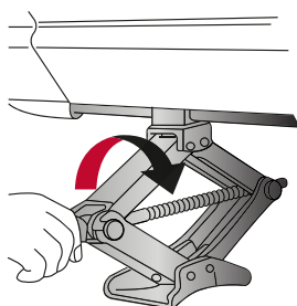
GIRE com as mãos
