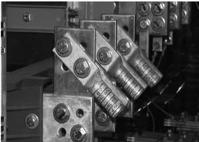
Figure 19. Lug adapters
