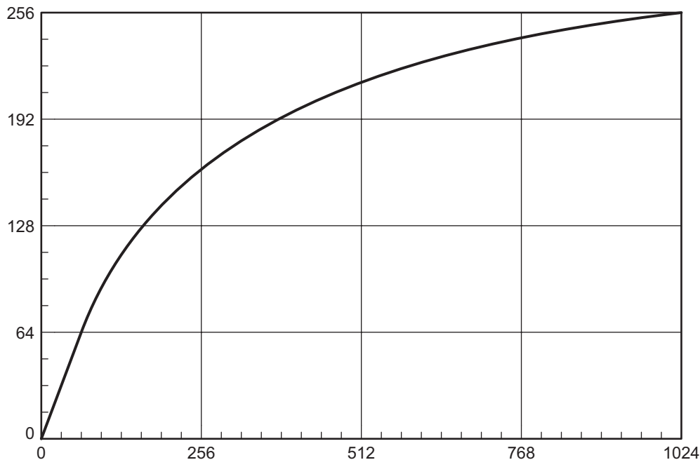
Figure 28. A-Law Table
