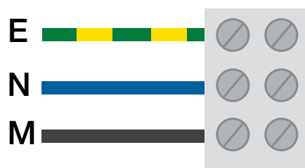
Slave conversion wiring: Switched live (L), Neutral (N), Earth (E)
