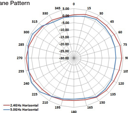
H-Plane Pattern
