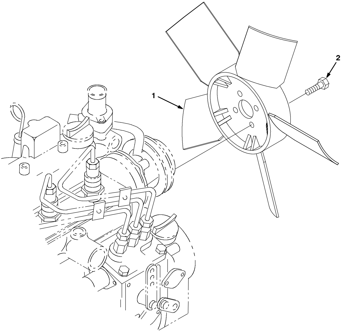
Fig. 28 - Fan Group
