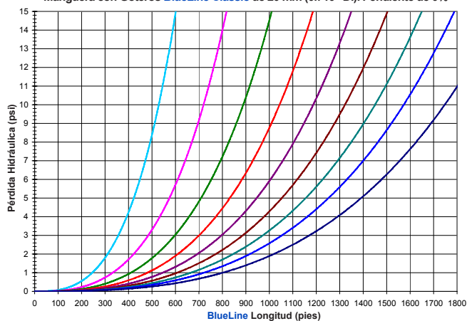
Pérdida Hidráulica vs. Longitud y Espaciamento entre goteros: Manguera con Goteros BlueLine Classic de 20 mm (0.710" DI). Pendiente de 0%
