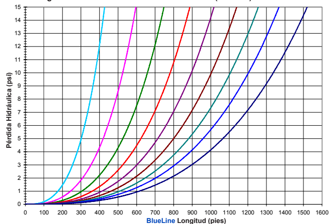
Pérdida Hidráulica vs. Longitud y Espaciamento entre goteros: Manguera con Goteros BlueLine Classic de 18 mm (0.620" DI). Pendiente de 0%
