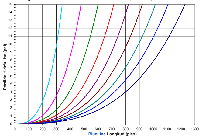
Pérdida Hidráulica vs. Longitud y Espaciamento entre goteros: Manguera con Goteros BlueLine Classic de 16 mm (0.550" DI). Pendiente de 0%
