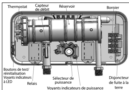
Figure 19 - Détail des composants du chauffe-eau
