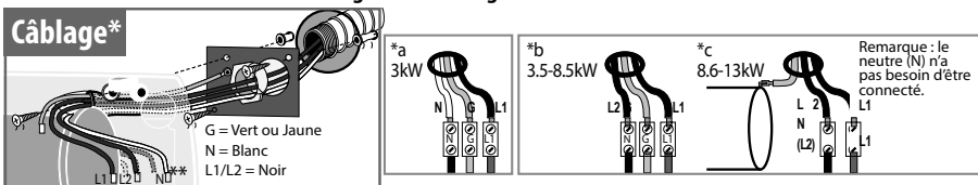
Figure 25 - Détail du câblage du chauffe-eau
