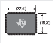
128-pin PEU (LQFP)
