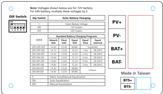
La Fig. 5.2. La bue arrière du SCC-30AB
