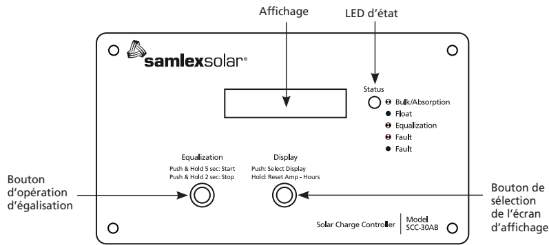
La Fig. 5.1. La plaque Frontale du SCC-30AB
