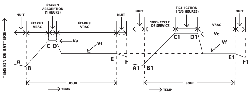
Fig.4.2A. Algorithme de charge normale
