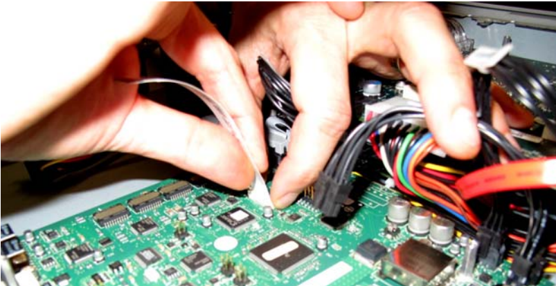
Figure 51: Attach Flex cable to AMB
